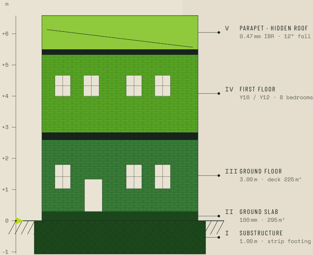
SECTION A-A · DOUBLE-STOREY VILLA · SCALE 1:100
