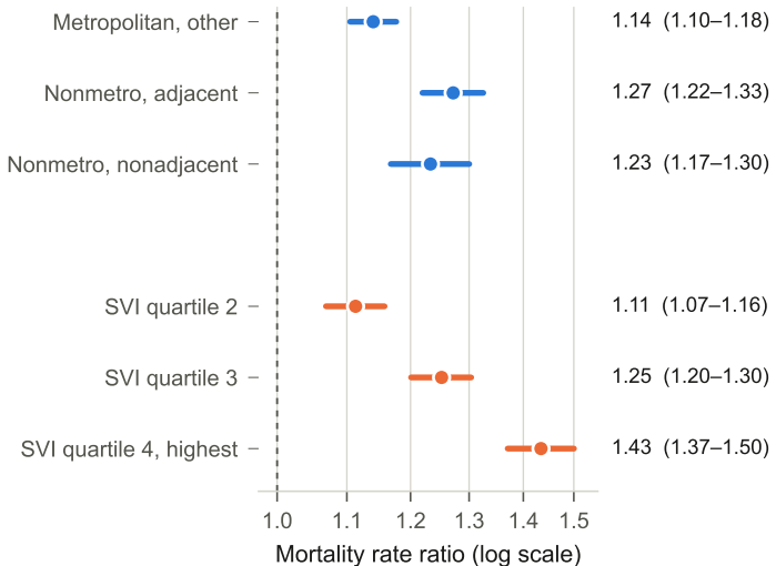
a Posterior rate ratios
