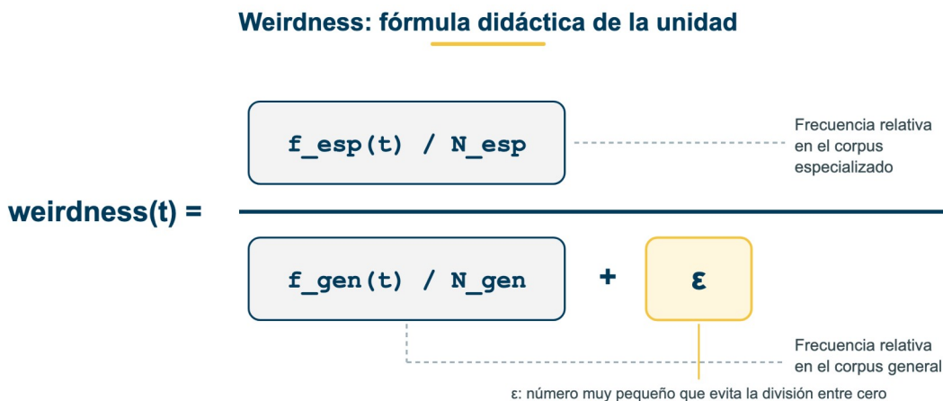
Figura 2. Componentes de la fórmula de weirdness
