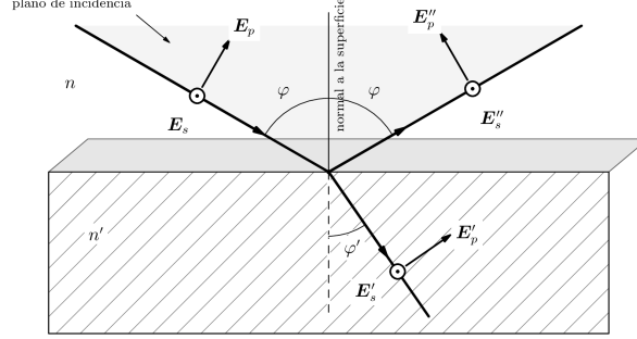
Figura 2.1: Descomposición del campo eléctrico en las polarizaciones s y p en una interfaz plana entre dos medios de índices n y n' . La componente \mathbf{E}_s es perpendicular al plano de incidencia (sale del dibujo), y la componente \mathbf{E}_p yace en él; cada onda (incidente, reflejada y transmitida) lleva su propio par (\mathbf{E}_s, \mathbf{E}_p) .
