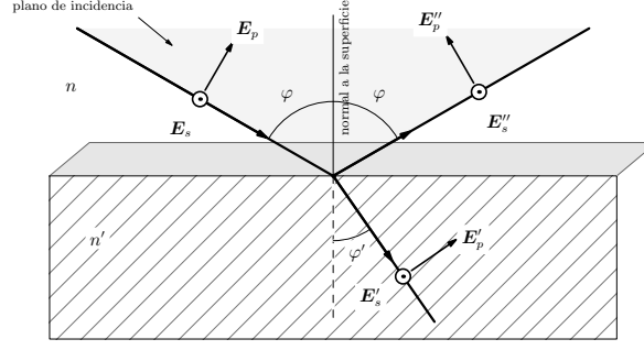
Figura 2.1: Descomposición del campo eléctrico en las polarizaciones s y p en una interfaz plana entre dos medios de índices n y n' . La componente \mathbf{E}_s es perpendicular al plano de incidencia (sale del dibujo), y la componente \mathbf{E}_p yace en él; cada onda (incidente, reflejada y transmitida) lleva su propio par (\mathbf{E}_s, \mathbf{E}_p) .
