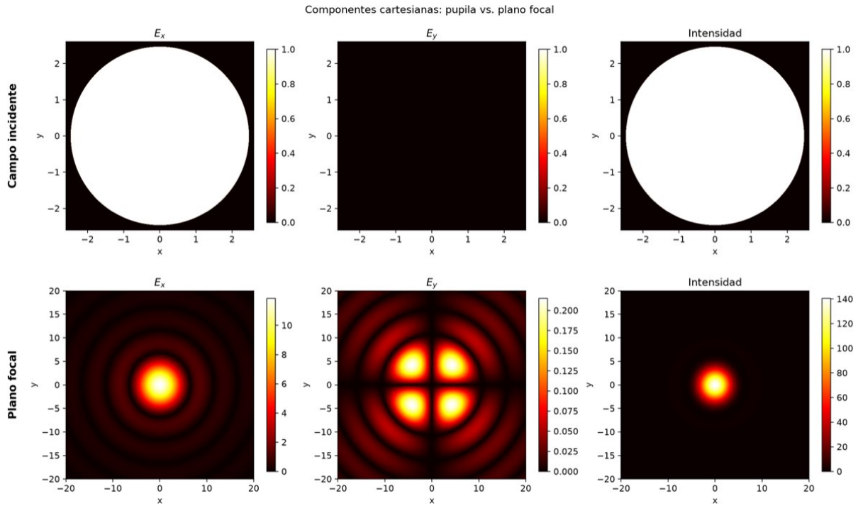
Figura III.11: Componentes cartesianas |E_x| , |E_y| e intensidad para incidencia lineal \hat{\mathbf{x}} : campo sobre la pupila (fila superior) y campo en el plano focal (fila inferior). Dioptrio estigmático con n_0 = 1 , n_i = 1.5 , z_0 = -10 mm, z_i = 6 mm, \lambda = 532 nm y pupila uniforme. La componente |E'_y| corresponde a la polarización cruzada, con el patrón de cuatro lóbulos \sin 2\varphi predicho por (III.176).
