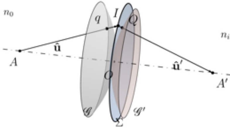
Figura III.1: Esferas de referencia \mathcal{G} y \mathcal{G}' . \mathcal{G} está centrada en el punto objeto A y \mathcal{G}' en el punto imagen A' ; ambas son tangentes al dioptrio en el vértice. El campo \mathbb{E}^{\mathcal{G}} es la amplitud incidente sobre \mathcal{G} , y \mathbb{E}^{\mathcal{G}'} es el campo transmitido sobre \mathcal{G}' , sobre el que la fase es constante por la condición estigmática.
