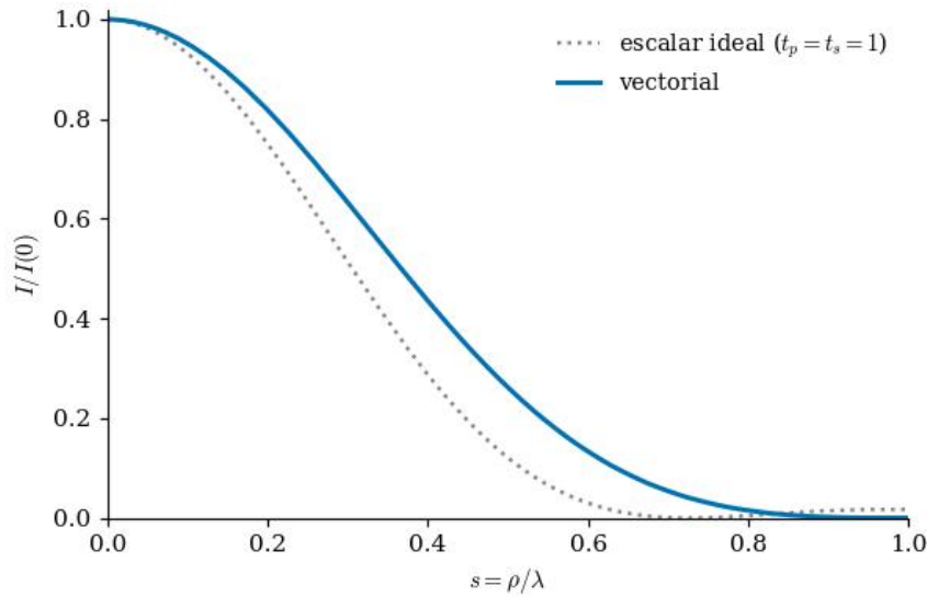
Figura III.14: Corte radial de la intensidad en el plano focal para incidencia lineal en el dioptrio de vidrio ( n_0 = 1 , n_i = 1.5 , z_0 = -10 mm, z_i = 6 mm, \lambda = 532 nm, pupila uniforme a apertura alta). La transmisión vectorial de Fresnel ensancha el punto focal respecto de la referencia escalar ideal ( t_p = t_s = 1 ); a esta escala los cortes por los dos ejes principales son indistinguibles.
