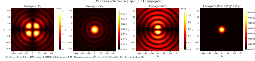
Figure III.12: Campo propagado en la base cartesiana para la condición inicial \mathcal{E}_{\perp,0} = (0, 1)^T .
