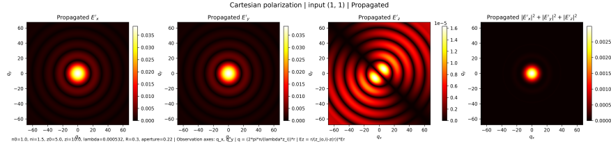
Figure III.13: Campo propagado en la base cartesiana para la condición inicial \mathcal{E}_{\perp,0} = (1, 1)^T .
