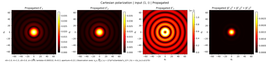
Figure III.14: Campo propagado en la base cartesiana para la condición inicial \mathcal{E}_{\perp,0} = (1, i)^T .
