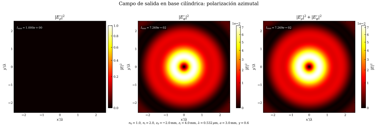
Figure III.11: Campo en el plano focal para incidencia azimutal, representado en base cilíndrica.
