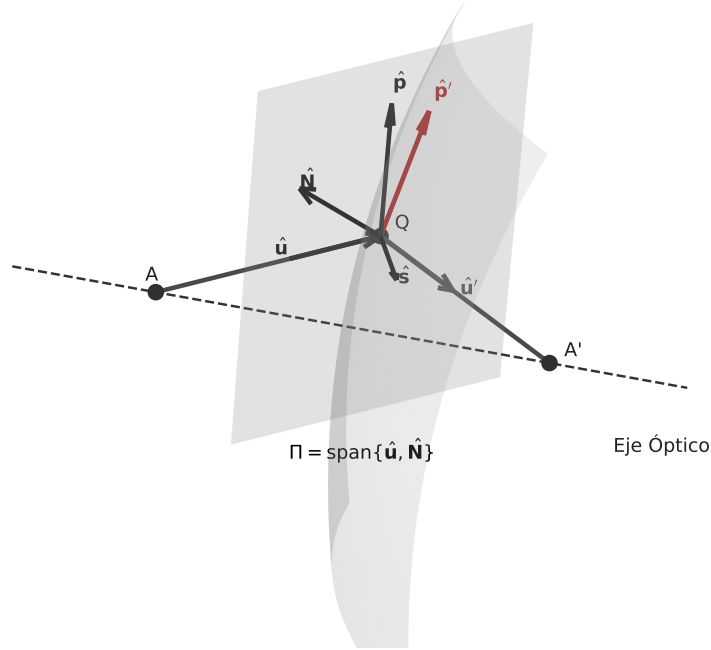
Figura II.3: Base de Fresnel en un punto Q de la interfaz refractante. El plano de incidencia \Pi = \text{span}\{\hat{\mathbf{u}}, \hat{\mathbf{N}}\} contiene la normal \hat{\mathbf{N}} y la dirección de propagación incidente \hat{\mathbf{u}} ; el vector \hat{\mathbf{p}} (y su homólogo transmitido \hat{\mathbf{p}}' ) yace en \Pi perpendicular a \hat{\mathbf{u}} (resp. \hat{\mathbf{u}}' ), mientras que \hat{\mathbf{s}} es perpendicular a \Pi .
