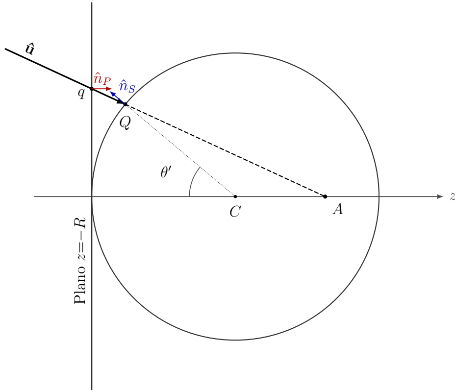
Figure A.1: Proyección al plano tangente con z horizontal y uso de \theta' \in [0, \pi/2] ( \theta = \pi - \theta' ). El rayo llega desde el exterior (línea continua) hasta Q y se prolonga (línea discontinua) hacia A = R(n_0/n_i) . El plano z = -R es la recta vertical a la izquierda.
