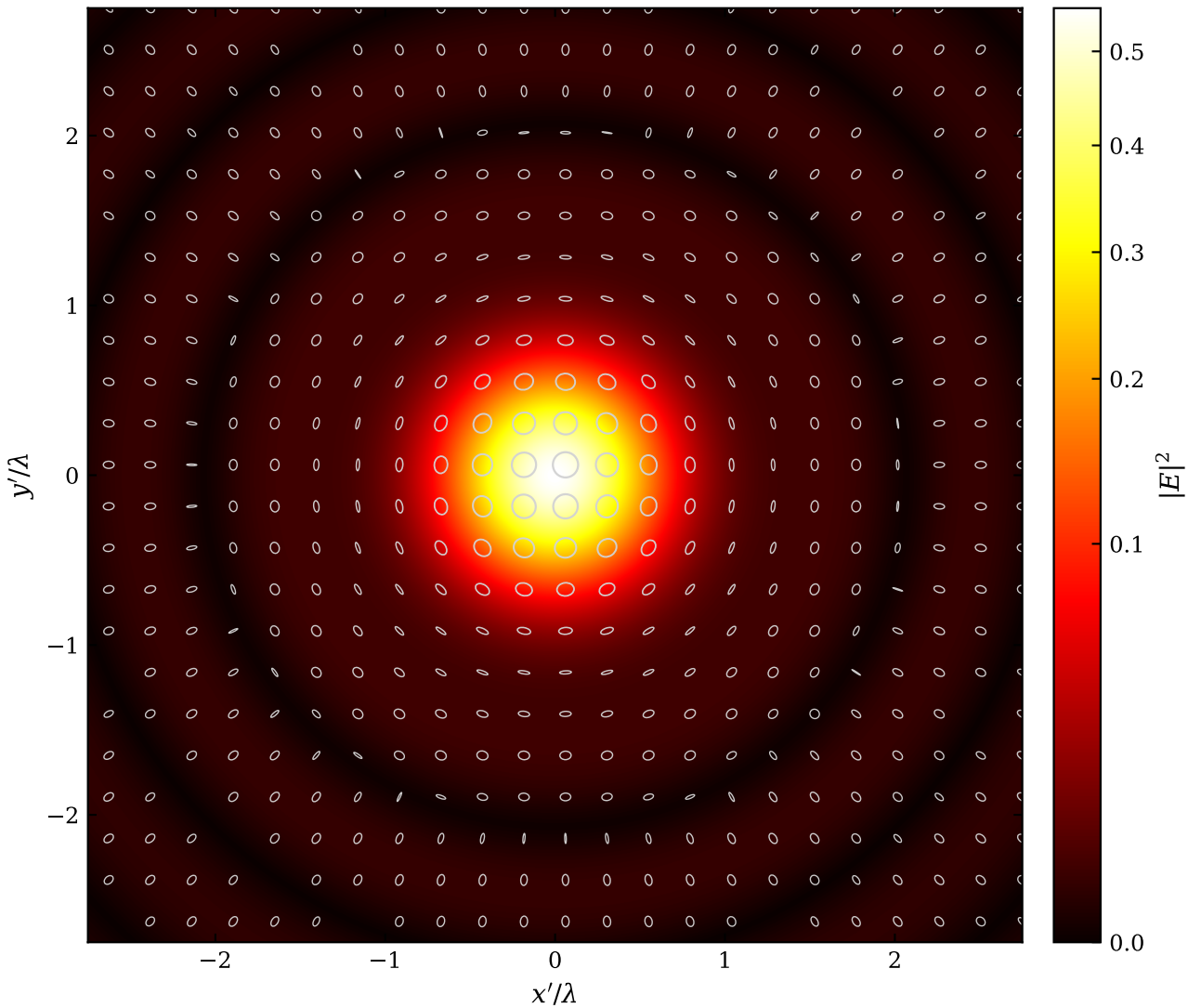
Mapa de polarización en el plano focal: incidencia circular
