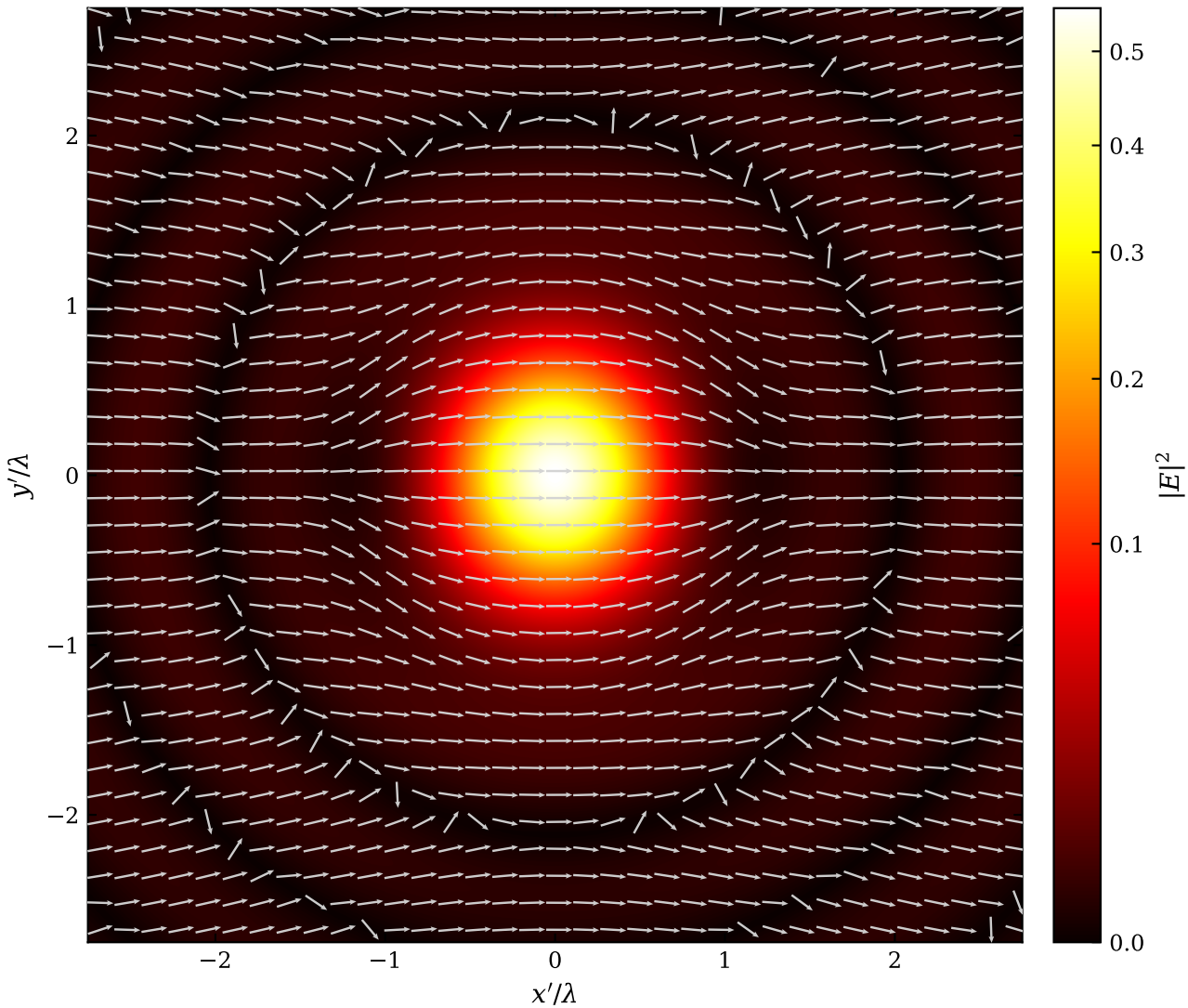
Mapa de polarización en el plano focal: incidencia lineal
