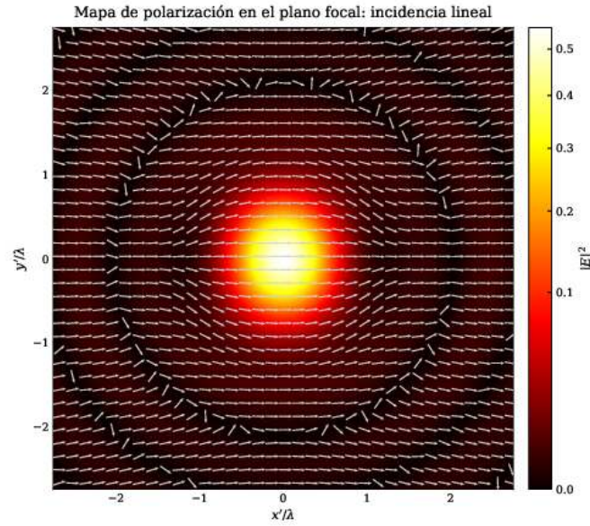
Figure III.14: Mapa de polarización en el plano focal para incidencia lineal. El fondo muestra |E|^2 y las flechas la orientación local, evidenciando la rotación inducida por la componente cruzada.
