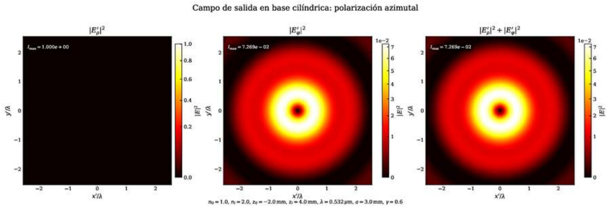
Figure III.12: Campo en el plano focal para incidencia azimutal, representado en base cilíndrica.
