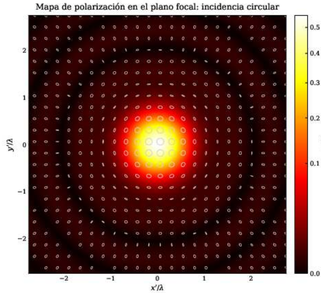
Figure III.4: Mapa de polarización en el plano focal para incidencia circular. El fondo muestra |E|^2 y las elipses la polarización local, incluyendo la modificación espacial de la helicidad.
