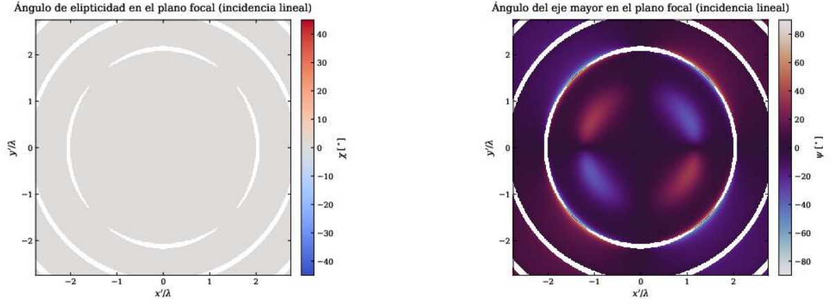
Figure III.15: Mapas escalares en el plano focal para incidencia lineal: ángulo de elipticidad \chi (izquierda) y ángulo del eje mayor \psi (derecha). Las regiones en blanco corresponden a zonas de intensidad demasiado baja, donde estos parámetros dejan de estar bien definidos.
