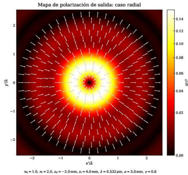
Figure III.8: Mapa de polarización en el plano focal para incidencia radial, con muestreo polar y centro excluido.
