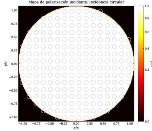
Figure III.3: Mapa de polarización del campo incidente circular. El fondo muestra |E|^2 y las elipses el estado local de polarización.
