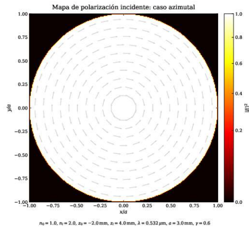
Figure III.10: Mapa de polarización del campo incidente azimutal. El centro se excluye por la singularidad de la base cilíndrica.
