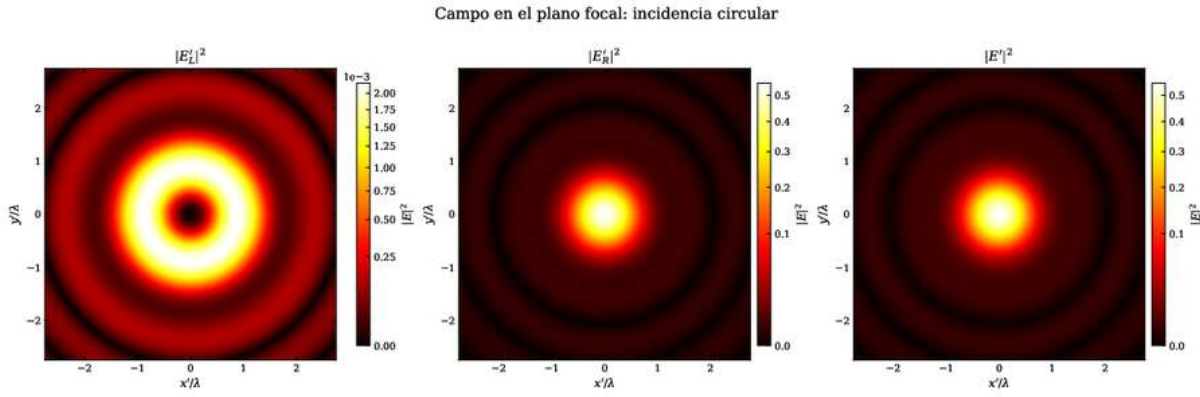
Figure III.6: Campo en el plano focal para incidencia circular. La componente opuesta representa la conversión parcial de helicidad.
