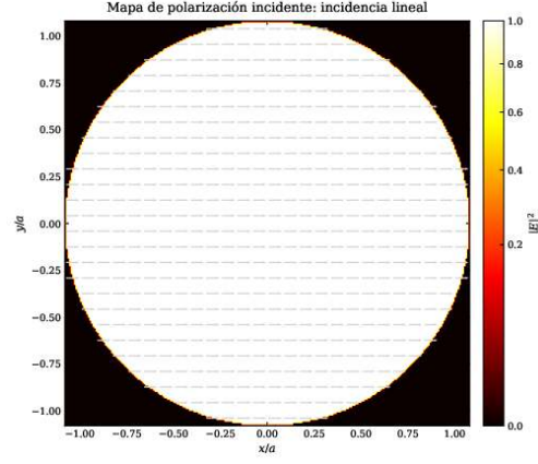
Figure III.13: Mapa de polarización del campo incidente lineal. El fondo muestra |E|^2 y las flechas la orientación local de la polarización.
