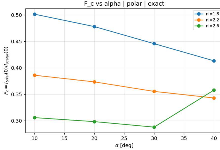
Figure III.17: F_c = I_{\text{total}}(0)/I_{\text{escalar}}(0) en función del ángulo de semiapertura \alpha para tres valores del índice de refracción del medio imagen n_i , con polarización cilíndrica y modelo exacto ( \lambda = 532 nm).
