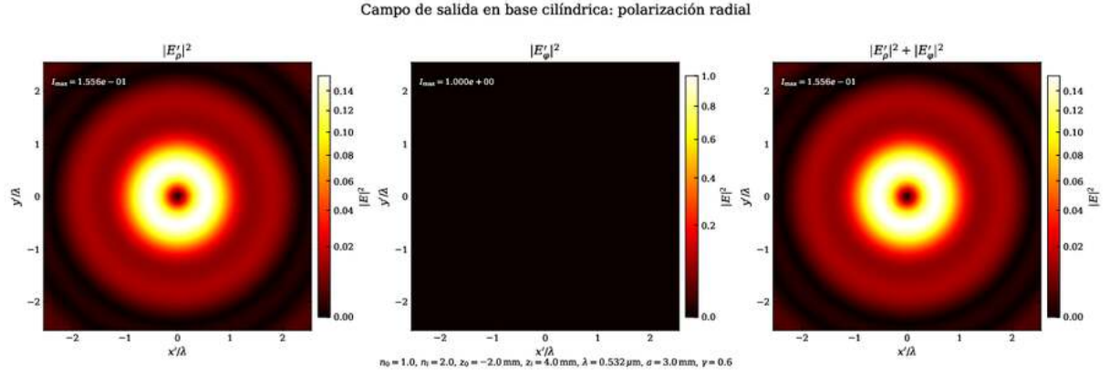
Figure III.9: Campo en el plano focal para incidencia radial, representado en base cilíndrica.
