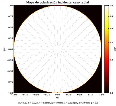
Figure III.7: Mapa de polarización del campo incidente radial. El centro se excluye por la singularidad de la base cilíndrica.
