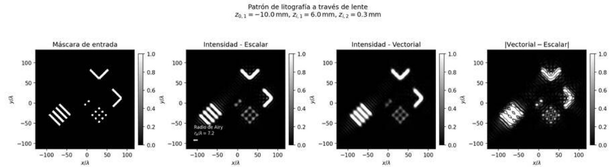
Figure III.2: Formación de un patrón litográfico para un campo incidente sin simetría axial. De izquierda a derecha: máscara de entrada, intensidad predicha por el modelo escalar, intensidad predicha por el modelo vectorial y diferencia absoluta entre ambas.
