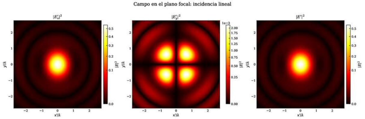
Figure III.16: Campo en el plano focal para incidencia lineal. La componente |E'_y|^2 corresponde a la polarización cruzada.
