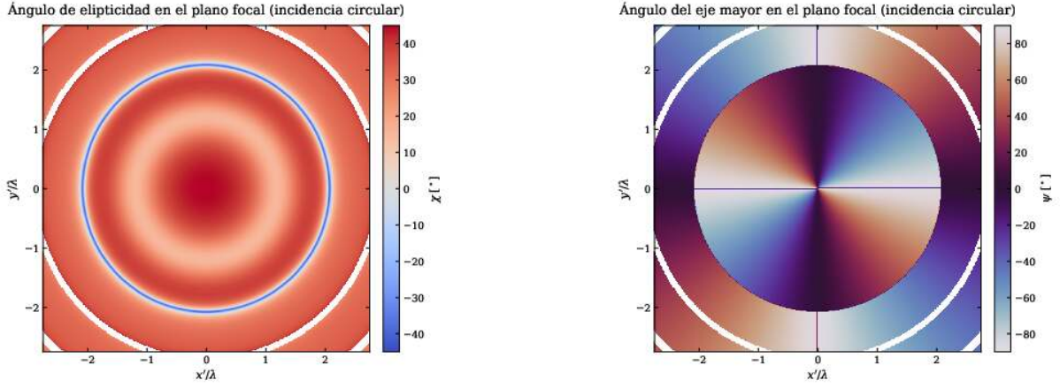
Figure III.5: Mapas escalares en el plano focal para incidencia circular: ángulo de elipticidad \chi (izquierda) y ángulo del eje mayor \psi (derecha). Las regiones en blanco corresponden a zonas de intensidad demasiado baja, donde estos parámetros dejan de estar bien definidos.
