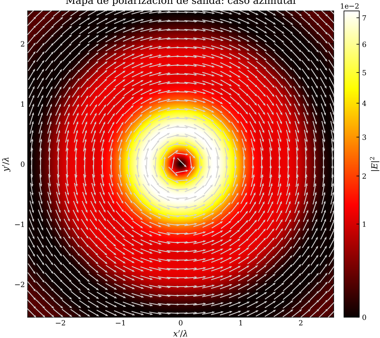
Mapa de polarización de salida: caso azimutal
