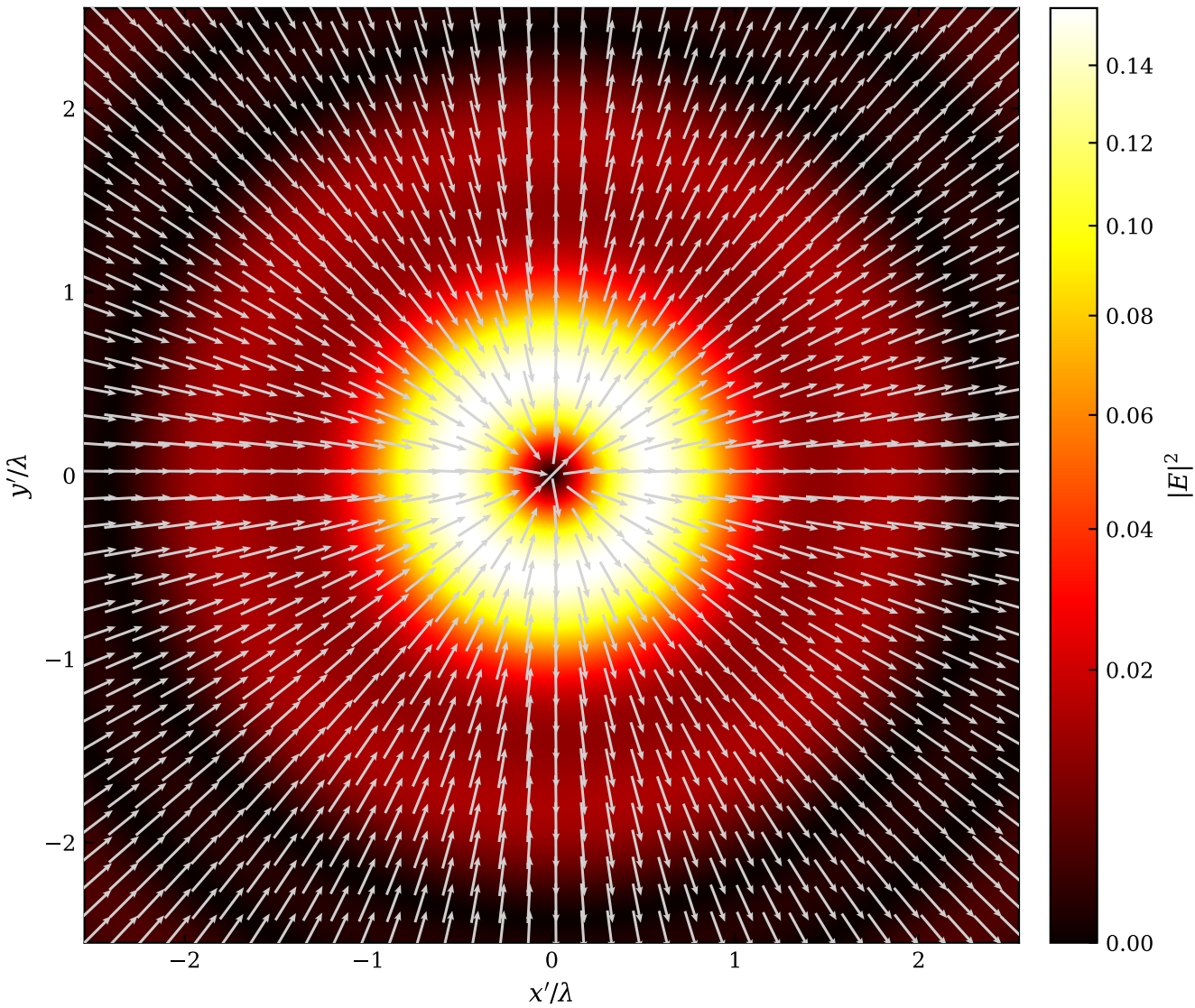
Mapa de polarización de salida: caso radial
