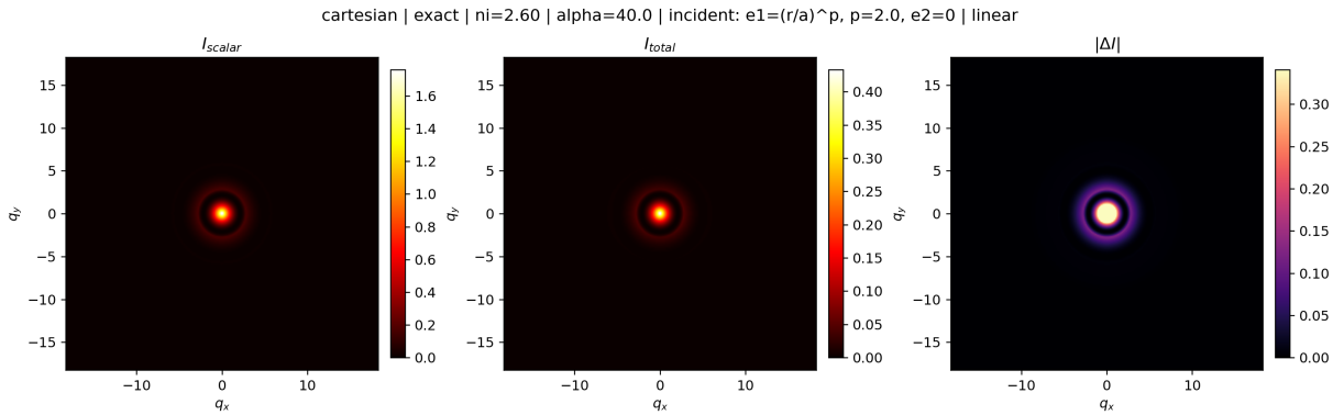
Figure III.15: Comparación de intensidades para polarización cartesiana, modelo exacto ( n_i = 2.6 , \alpha = 40^\circ ). La supresión central en I_{\text{total}} respecto de I_{\text{escalar}} refleja el mismo efecto que en la representación circular: la parte anisotrópica \mathcal{H}_2 redistribuye energía desde el centro hacia el entorno azimutal de orden dos.
