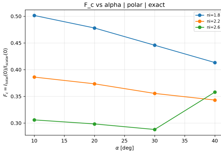
Figure III.16: F_c = I_{\text{total}}(0)/I_{\text{escalar}}(0) en función del ángulo de semiapertura \alpha para tres valores del índice de refracción del medio imagen n_i , con polarización cilíndrica y modelo exacto ( \lambda = 532 nm).
