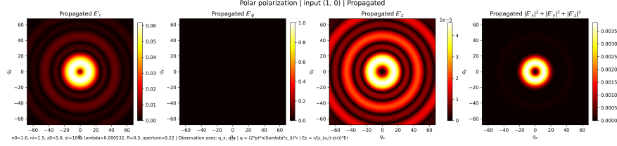
Figure III.6: Base cilíndrica, caso (1, 0): campo radialmente polarizado propagado.
