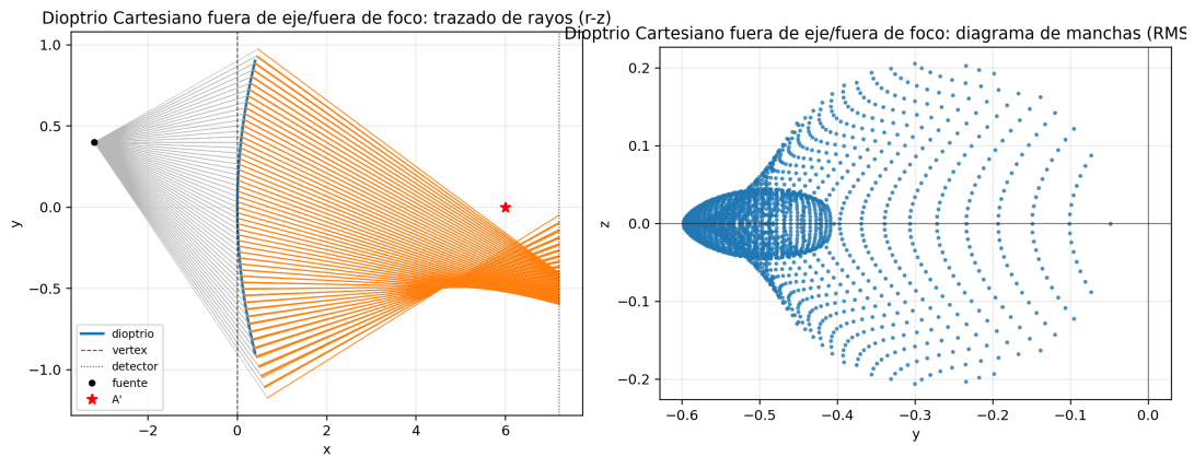
Figure I.4: Dioptrio cartesiano en condición fuera de eje y fuera de foco: el trazado en r - z y el spot diagram muestran pérdida de concentración al romperse la condición conjugada nominal.
