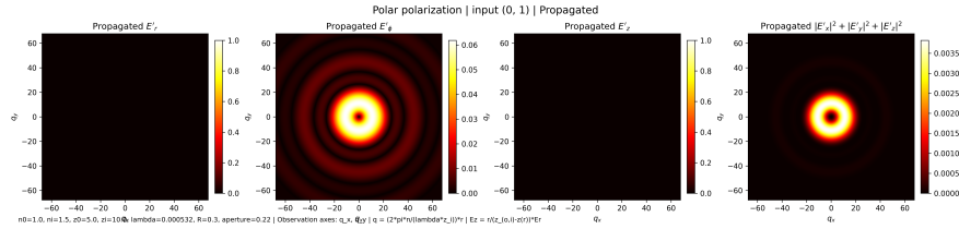
Figure III.7: Base cilíndrica, caso (0, 1): campo azimutalmente polarizado propagado.
