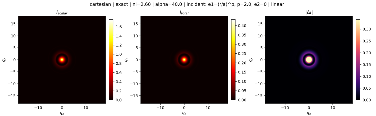
Figure III.15: Comparación de intensidades para polarización cartesiana, modelo exacto ( n_i = 2.6 , \alpha = 40 ). La supresión central en I_{\text{total}} respecto de I_{\text{escalar}} refleja el mismo efecto que en la representación circular: la parte anisotrópica \mathcal{H}_2 redistribuye energía desde el centro hacia el entorno azimutal de orden dos.
