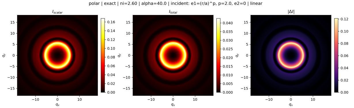
Figure III.10: Comparación de intensidades para polarización cilíndrica, modelo exacto ( n_i = 2.6 , \alpha = 40 ). La estructura anular de I_{\text{total}} confirma el cero axial predicho por la transformada de Hankel de orden uno para modos radial o azimutalmente polarizados con simetría azimutal.
