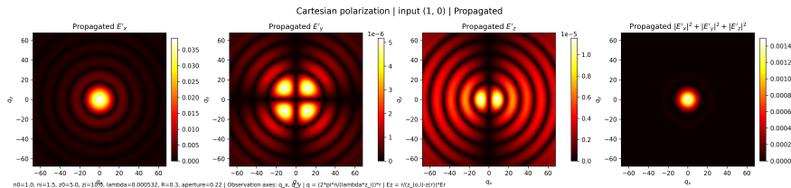
Figure III.11: Campo propagado en la base cartesiana para la condición inicial \mathcal{E}_{\perp,0} = (1, 0)^T .
