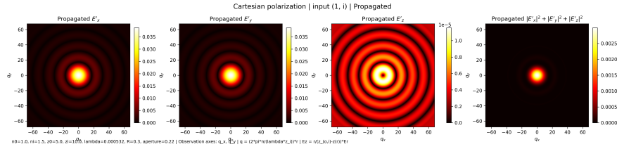
Figure III.14: Campo propagado en la base cartesiana para la condición inicial \mathcal{E}_{\perp,0} = (1, i)^T .
