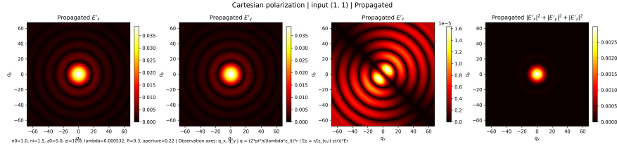
Figure III.13: Campo propagado en la base cartesiana para la condición inicial \mathcal{E}_{\perp,0} = (1, 1)^T .
