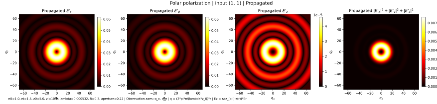
Figure III.8: Base cilíndrica, caso (1, 1): superposición radial-azimutal propagada.
