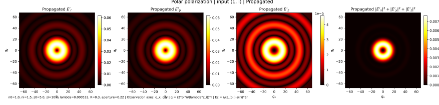
Figure III.9: Base cilíndrica, caso (1, i) : superposición radial–azimutal con desfase relativo propagada.
