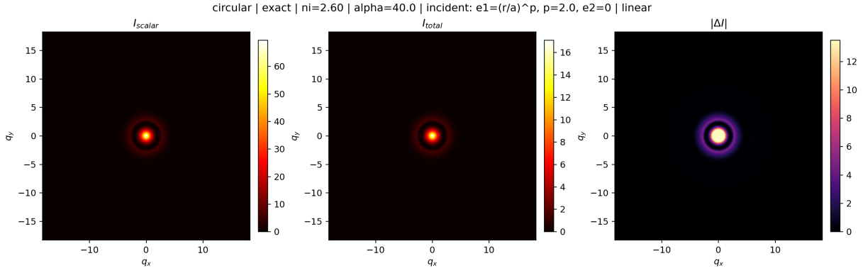
Figure III.5: Comparación de intensidades para polarización circular, modelo exacto ( n_i = 2.6 , \alpha = 40 ). De izquierda a derecha: intensidad escalar I_{escalar} , intensidad vectorial total I_{total} , y diferencia absoluta |\Delta I| . El centro del foco presenta la mayor discrepancia entre ambas descripciones.
