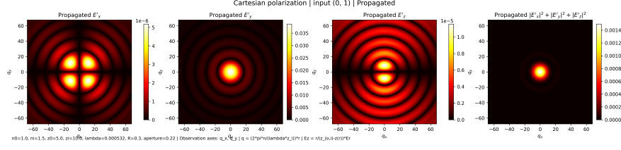
Figure III.12: Campo propagado en la base cartesiana para la condición inicial \mathcal{E}_{\perp,0} = (0, 1)^T .
