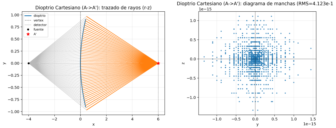
Figure I.1: Dioptrio cartesiano, fuente en A y detector en A' : en el corte r - z se observa convergencia al plano focal y un spot prácticamente puntual (RMS numéricamente cercano a cero).
