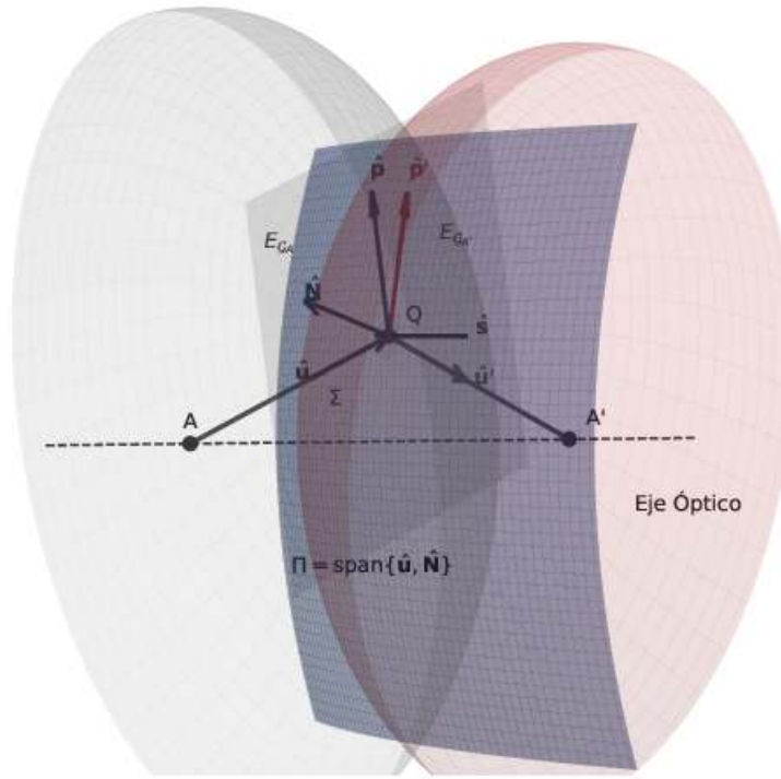
Figura III.1: Esferas de referencia \mathcal{G} y \mathcal{G}' . \mathcal{G} está centrada en el punto objeto A y \mathcal{G}' en el punto imagen A' ; ambas son tangentes al dioptrio en el vértice. El campo \mathbb{E}^{\mathcal{G}} es la amplitud incidente sobre \mathcal{G} , y \mathbb{E}^{\mathcal{G}'} es el campo transmitido sobre \mathcal{G}' , sobre el que la fase es constante por la condición estigmática.
