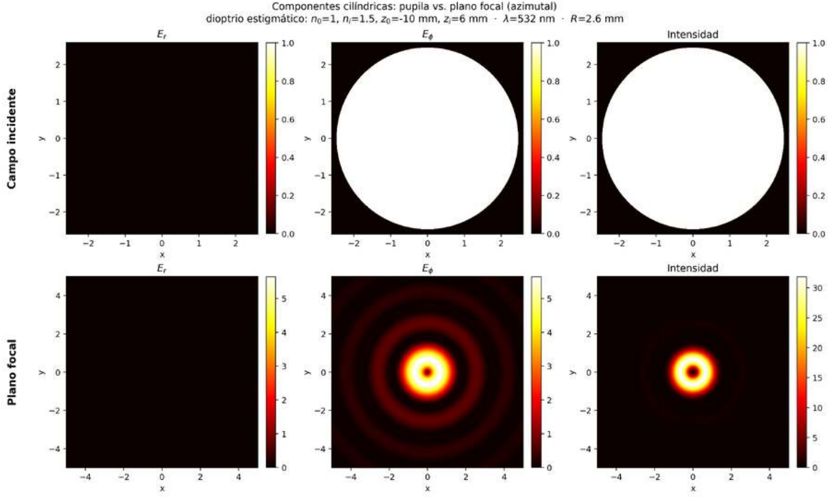
Figura III.9: Componentes cilíndricas |E_r| , |E_\phi| e intensidad para incidencia azimutal: campo sobre la pupila (fila superior) y campo en el plano focal (fila inferior), con los mismos parámetros de la figura III.7. La polarización azimutal es modo propio de la transmisión (coeficiente t_s ) y el plano focal exhibe de nuevo el anillo con centro oscuro.
