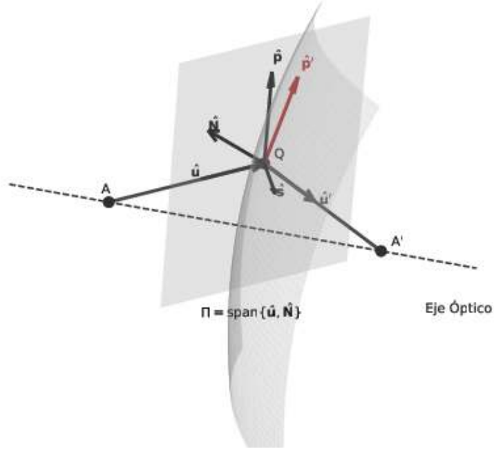
Figura II.3: Base de Fresnel en un punto Q de la interfaz refractante. El plano de incidencia \Pi = \text{span}\{\hat{u}, \hat{N}\} contiene la normal \hat{N} y la dirección de propagación incidente \hat{u} ; el vector \hat{p} (y su homólogo transmitido \hat{p}' ) yace en \Pi perpendicular a \hat{u} (resp. \hat{u}' ), mientras que \hat{s} es perpendicular a \Pi .
