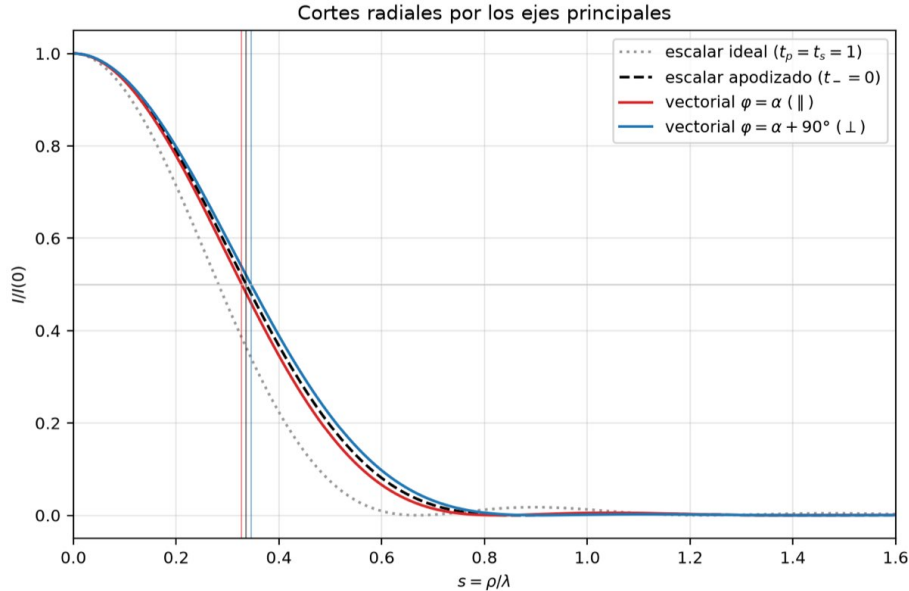
Figura III.14: Cortes de la intensidad focal por los ejes principales para incidencia lineal en el dioptrio de vidrio ( n_0 = 1 , n_i = 1.5 , z_0 = -10 mm, z_i = 6 mm, \lambda = 532 nm, pupila uniforme a apertura alta). El corte paralelo a la polarización se contrae y el perpendicular se expande respecto de la referencia escalar apodizada ( t_- = 0 ); la referencia escalar ideal ( t_p = t_s = 1 ) muestra que la apodización de Fresnel t_+(\rho') también ensancha el punto.
