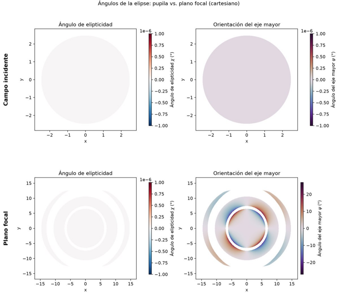
Figura III.13: Ángulos de la elipse de polarización para incidencia lineal \hat{\mathbf{x}} : elipticidad \chi (izquierda) y orientación del eje mayor \psi (derecha), sobre la pupila (fila superior) y en el plano focal (fila inferior). La elipticidad es nula en todo el plano focal: el estado permanece lineal y la aberración vectorial se reduce a una rotación local de la orientación. Las regiones en blanco corresponden a zonas de intensidad demasiado baja, donde estos parámetros dejan de estar bien definidos.
