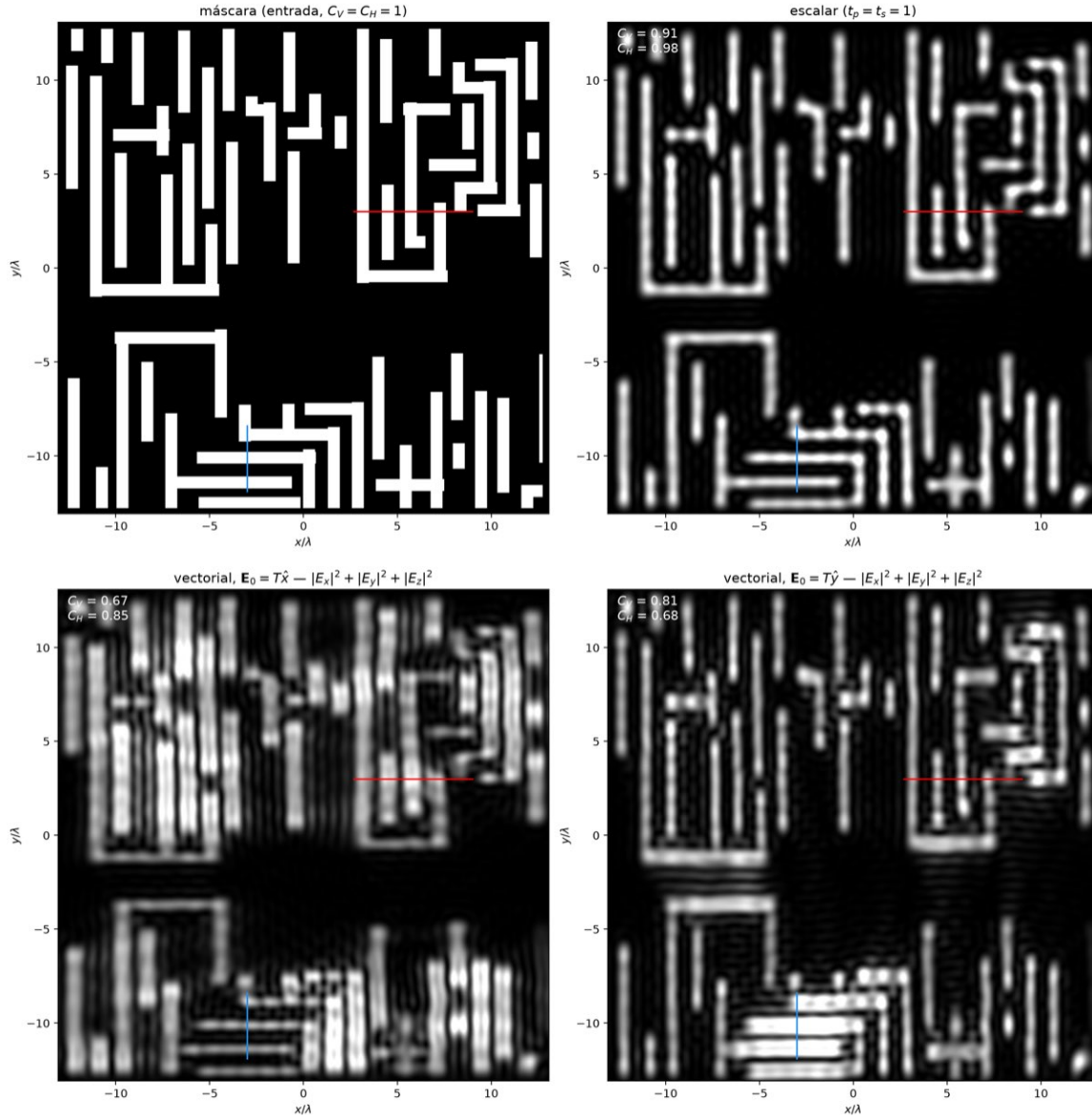
Figura III.2: Imagen de una máscara litográfica de tipo circuito formada por una lente de dos superficies cartesianas conjugadas ( \lambda = 193\text{ nm} , \text{NA} = 0.94 , aumento unitario, trazas de 0.64\lambda con paso fino de 1.23\lambda ). Arriba: máscara de entrada e intensidad predicha por el modelo escalar. Abajo: intensidad total del modelo vectorial para iluminación lineal \hat{x} (izquierda) y \hat{y} (derecha). En cada panel se indican los contrastes C_V y C_H medidos sobre los cortes señalados (rojo: trazas verticales; azul: trazas horizontales): las trazas alineadas con la polarización incidente se resuelven mejor que las ortogonales.
