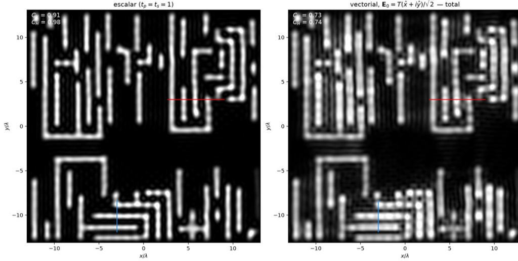
Figura III.3: Imagen del mismo patrón de la figura III.2 con iluminación circular: modelo escalar (izquierda) y vectorial con intensidad total (derecha). La pérdida de contraste se reparte por igual entre ambas orientaciones ( C_V = 0.73 , C_H = 0.74 ): la iluminación circular isotropiza la aberración vectorial, pero no la elimina.
