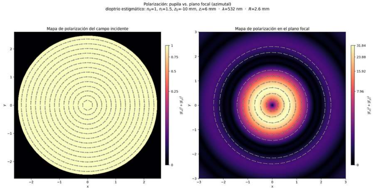
Figura III.10: Mapas de polarización para incidencia azimutal: campo sobre la pupila (izquierda) y campo en el plano focal (derecha). El estado local permanece azimutal punto a punto.
