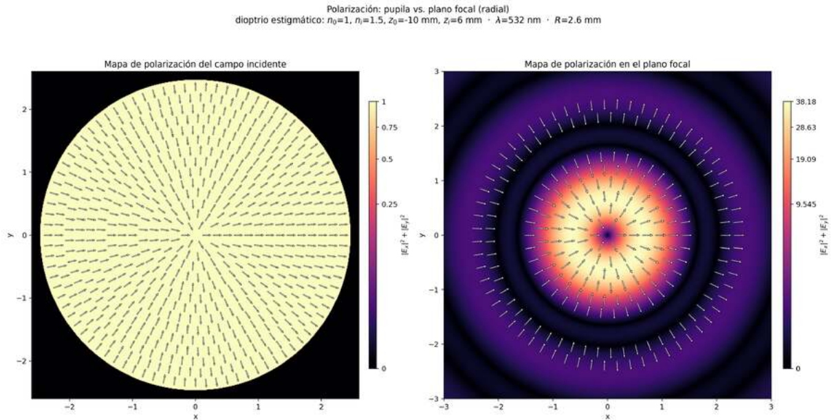
Figura III.8: Mapas de polarización para incidencia radial: campo sobre la pupila (izquierda) y campo en el plano focal (derecha). El fondo muestra |E_x|^2 + |E_y|^2 y los glifos el estado local de polarización, que permanece radial punto a punto.
