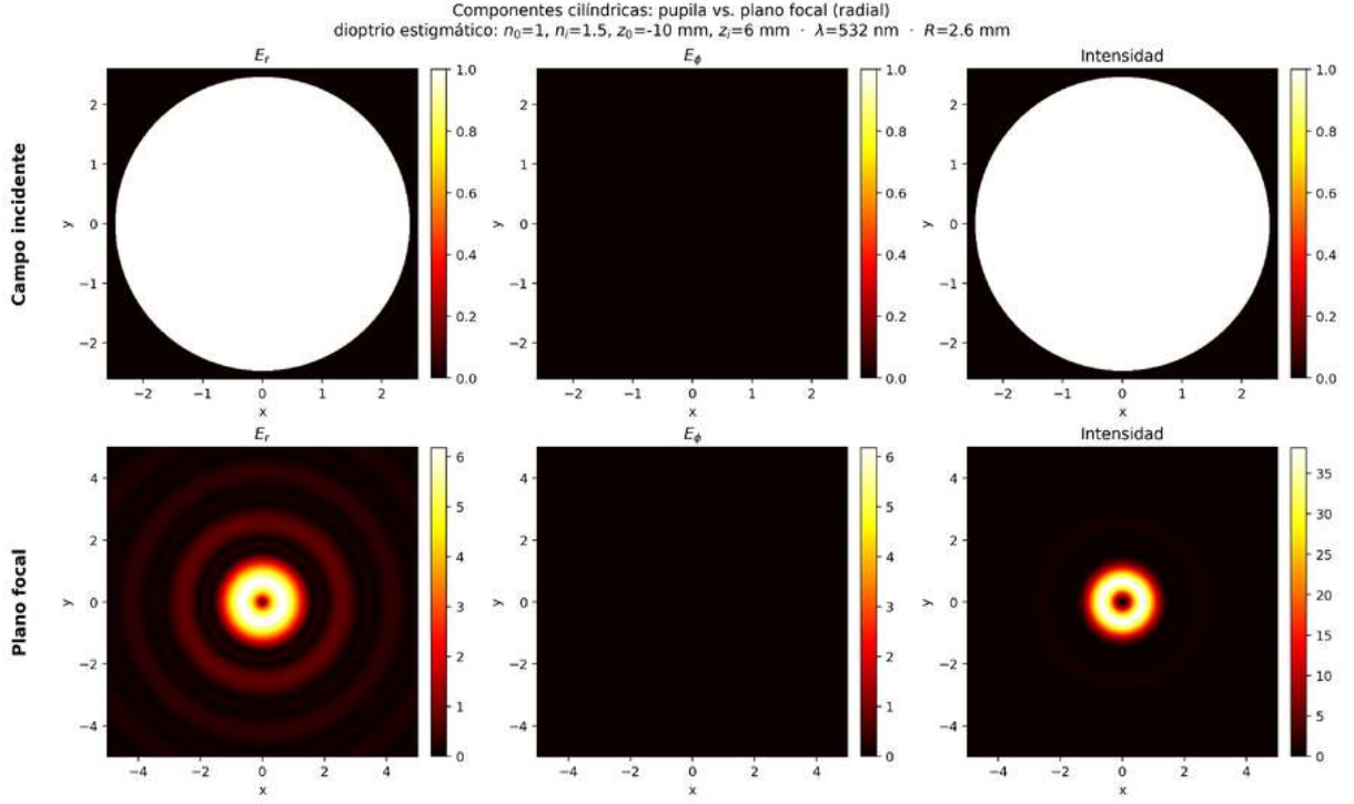
Figura III.7: Componentes cilíndricas |E_r| , |E_\phi| e intensidad para incidencia radial: campo sobre la pupila (fila superior) y campo en el plano focal (fila inferior). Dioptrio estigmático con n_0 = 1 , n_i = 1.5 , z_0 = -10 mm, z_i = 6 mm, \lambda = 532 nm y pupila uniforme. La transmisión es diagonal en esta base: no aparece componente azimutal, y la estructura de Hankel de orden uno produce el centro oscuro.
