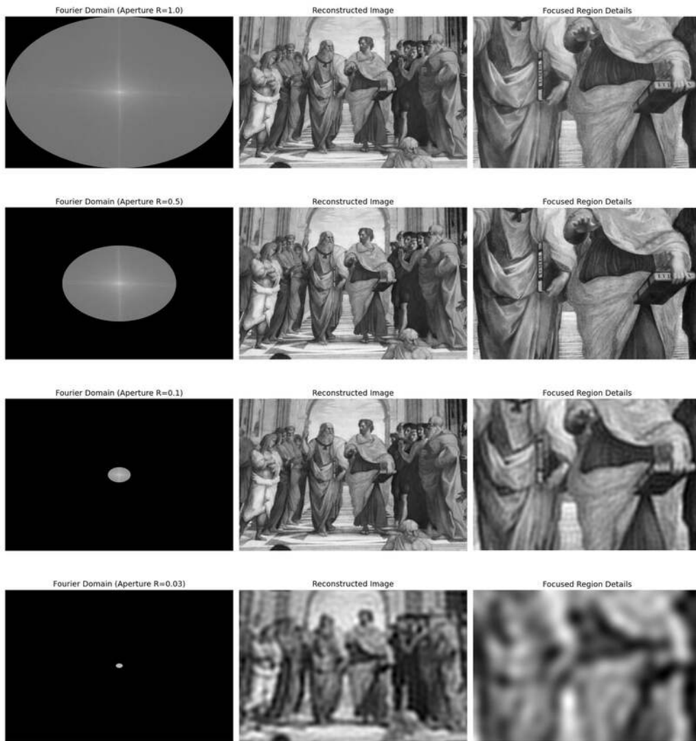
Figura II.2: Pérdida de detalle al reducir la apertura numérica: las frecuencias espaciales altas quedan fuera de banda y no son transmitidas por el sistema óptico. Se observa que las frecuencias espaciales más altas contienen los detalles más finos.
