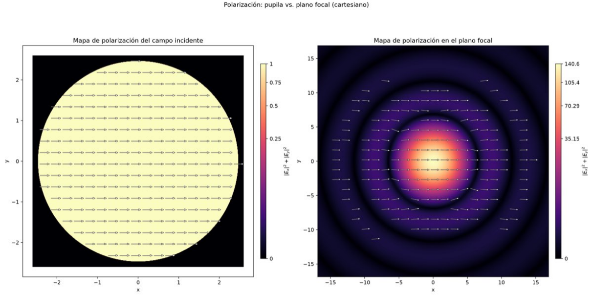
Figura III.12: Mapas de polarización para incidencia lineal \hat{\mathbf{x}} : campo sobre la pupila (izquierda) y campo en el plano focal (derecha). El fondo muestra |E_x|^2 + |E_y|^2 y las flechas la orientación local de la polarización, evidenciando la rotación inducida por la componente cruzada.
