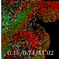
Ours
