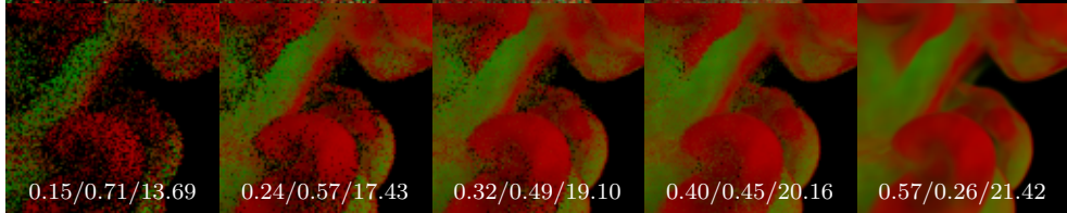
Ours
