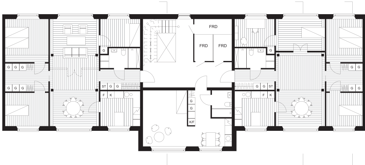
Plan 1-4, princip alt. 1 —Bostäder
