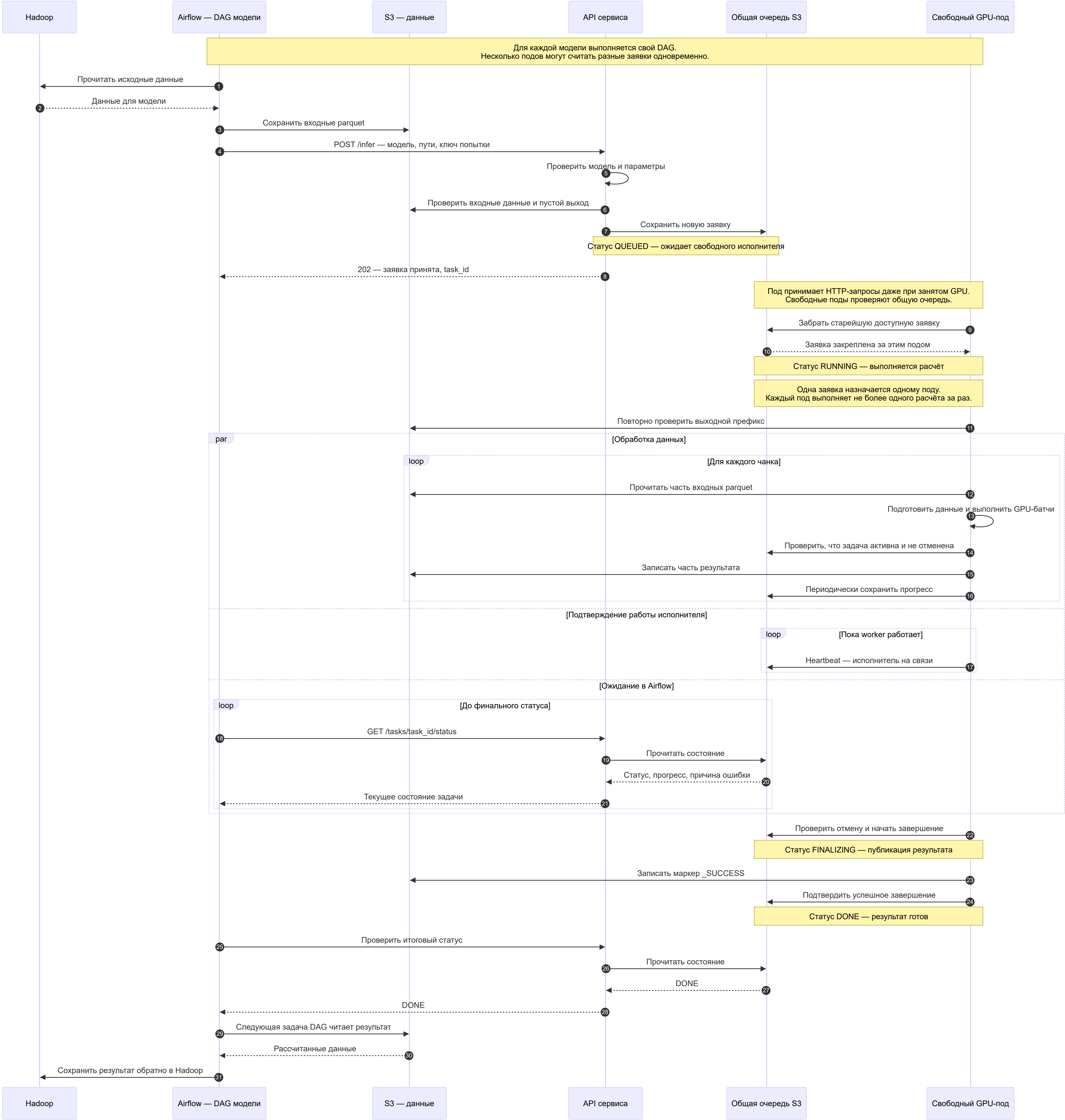
Успешный расчёт — UML sequence
