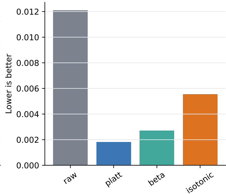
ECE
