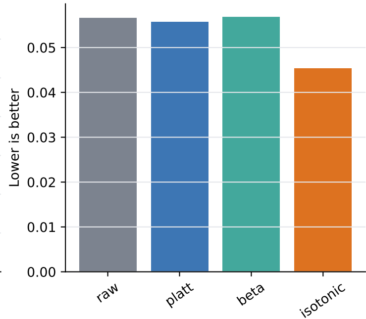
ECE
