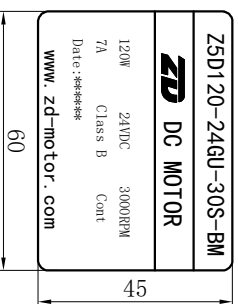
电机铭牌
