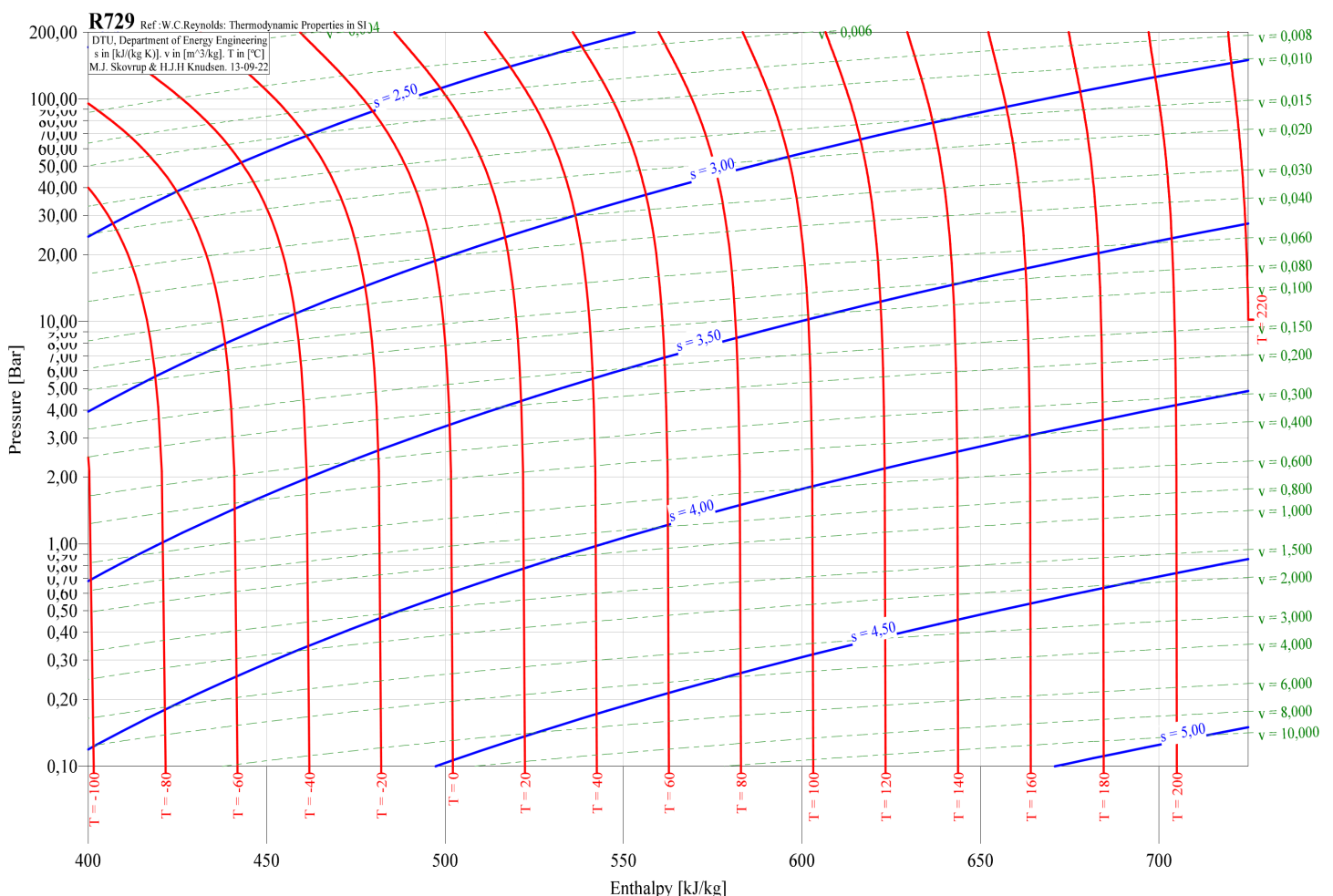
Fig. 12. – Diagramme (P,h) de l'air.
