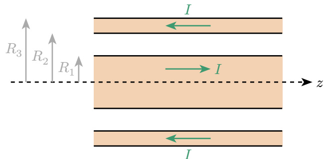
Coupe longitudinale
