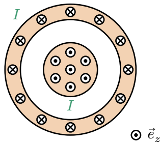
Coupe transversale
