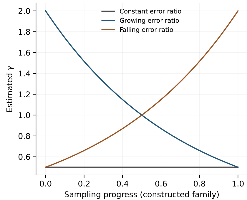
Compatible error hierarchies
