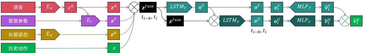
图 3.2 FaceCapGes 模型整体结构
