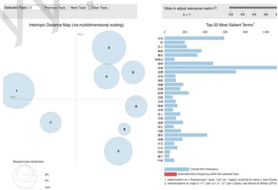
图 11：最佳主题 LDA 可视化图
