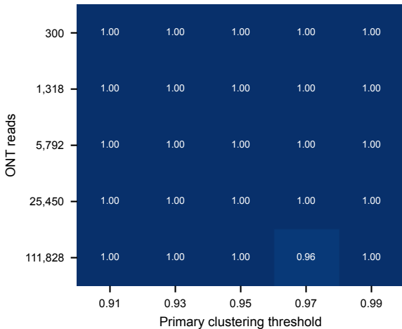
Precision
