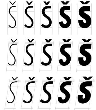
Scaron.ss04
