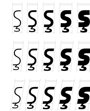
scedilla.ss03
