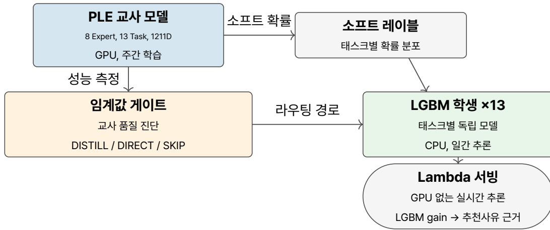
Figure 1: 교사-학생 종류 아키텍처.
