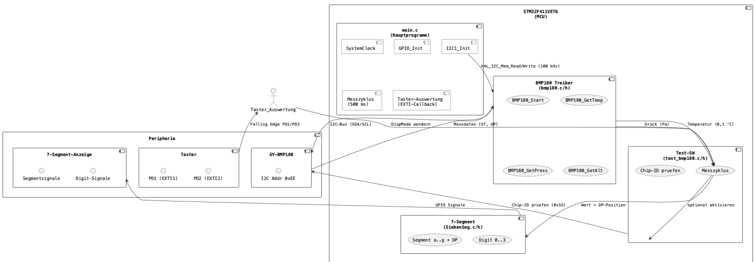
SysML IBD: Luftdruck-Sensor System Internal Block Diagram — Daten- und Signalflüsse
