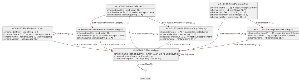
Abbildung 1: UML-Diagramm des Datenmodells von eCH-0265. Dieses Diagramm wurde automatisch mithilfe von SHACL PLAY! (Francart 2020) aus den SHACL-Spezifikationen generiert.
