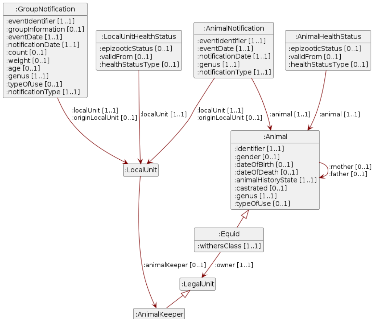
Abbildung 1: UML-Diagramm des Datenmodells von eCH-0309.
