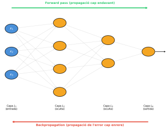
Figure 4: Lògica backpropagation
