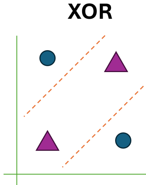
Figure 2: Problema XOR.
