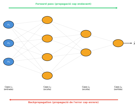
Figure 4: Lògica backpropagation
