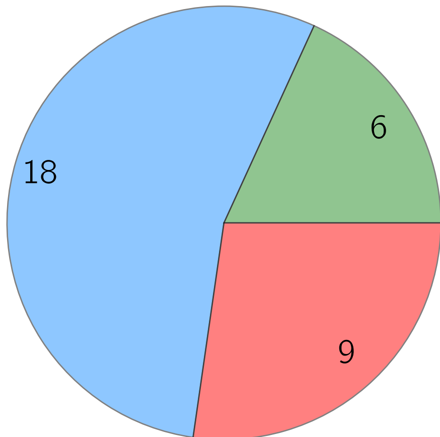
LOS Clouds
