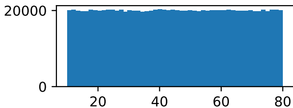
srcmass1
