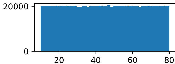
srcmass2
