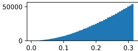
redshift
