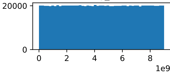
comoving_volume
