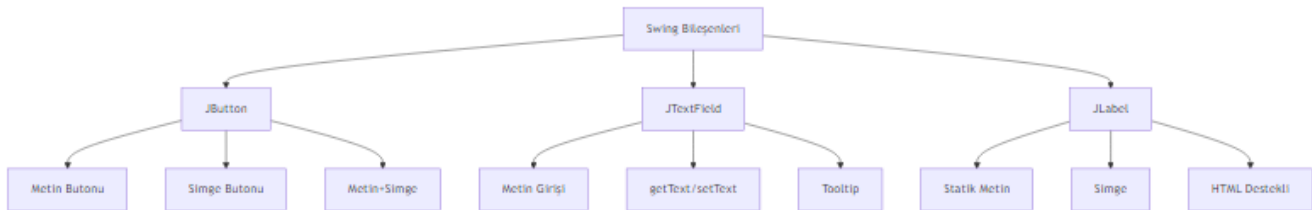
Şekil 31: Mermaid Diyagramı 37
