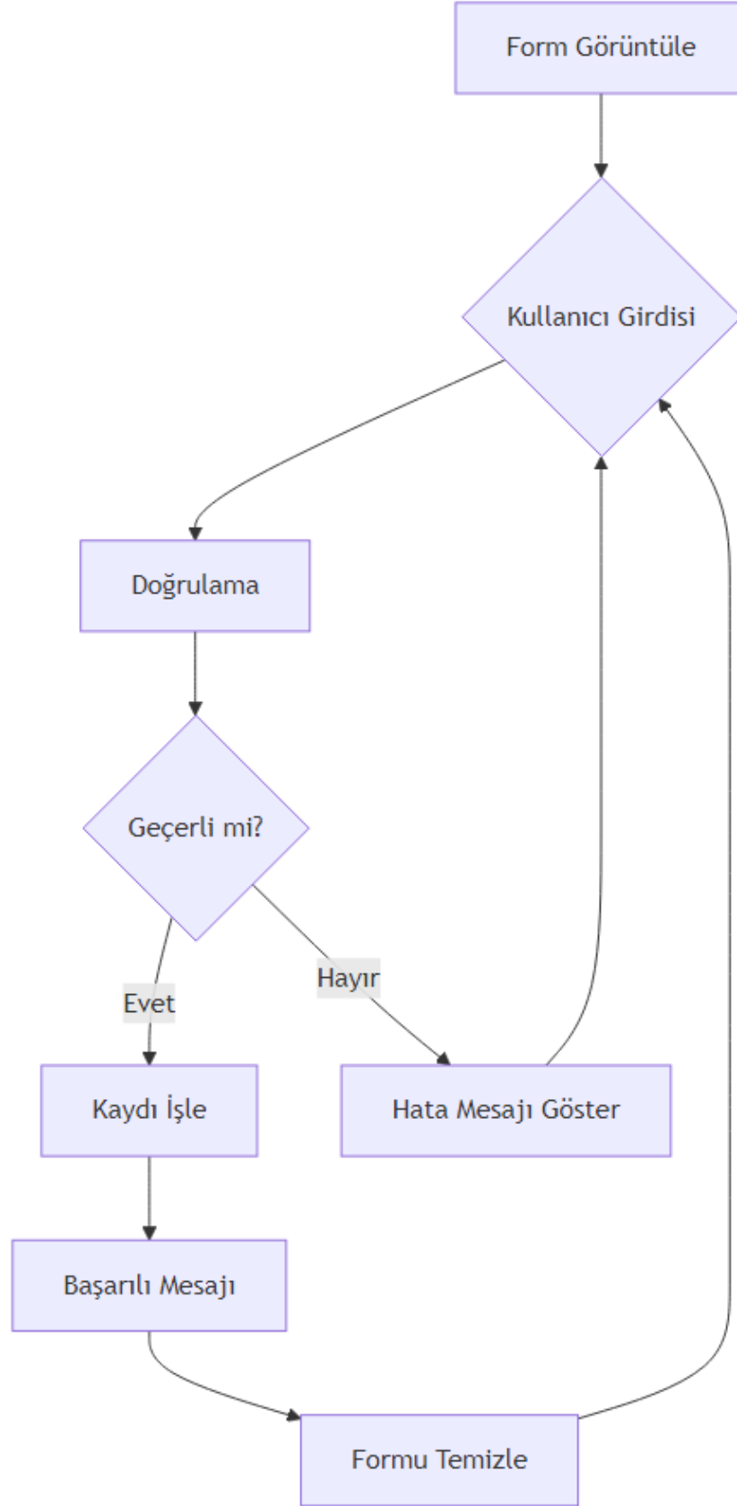
Şekil 33: Mermaid Diyagramı 39
