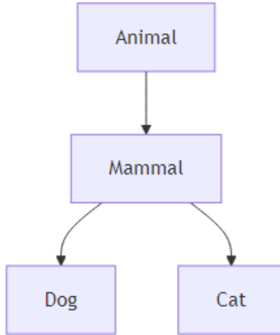
Şekil 24: Mermaid Diyagramı 29
