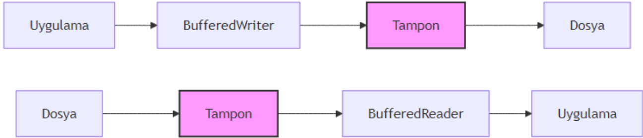
Şekil 19: Mermaid Diyagramı 23
