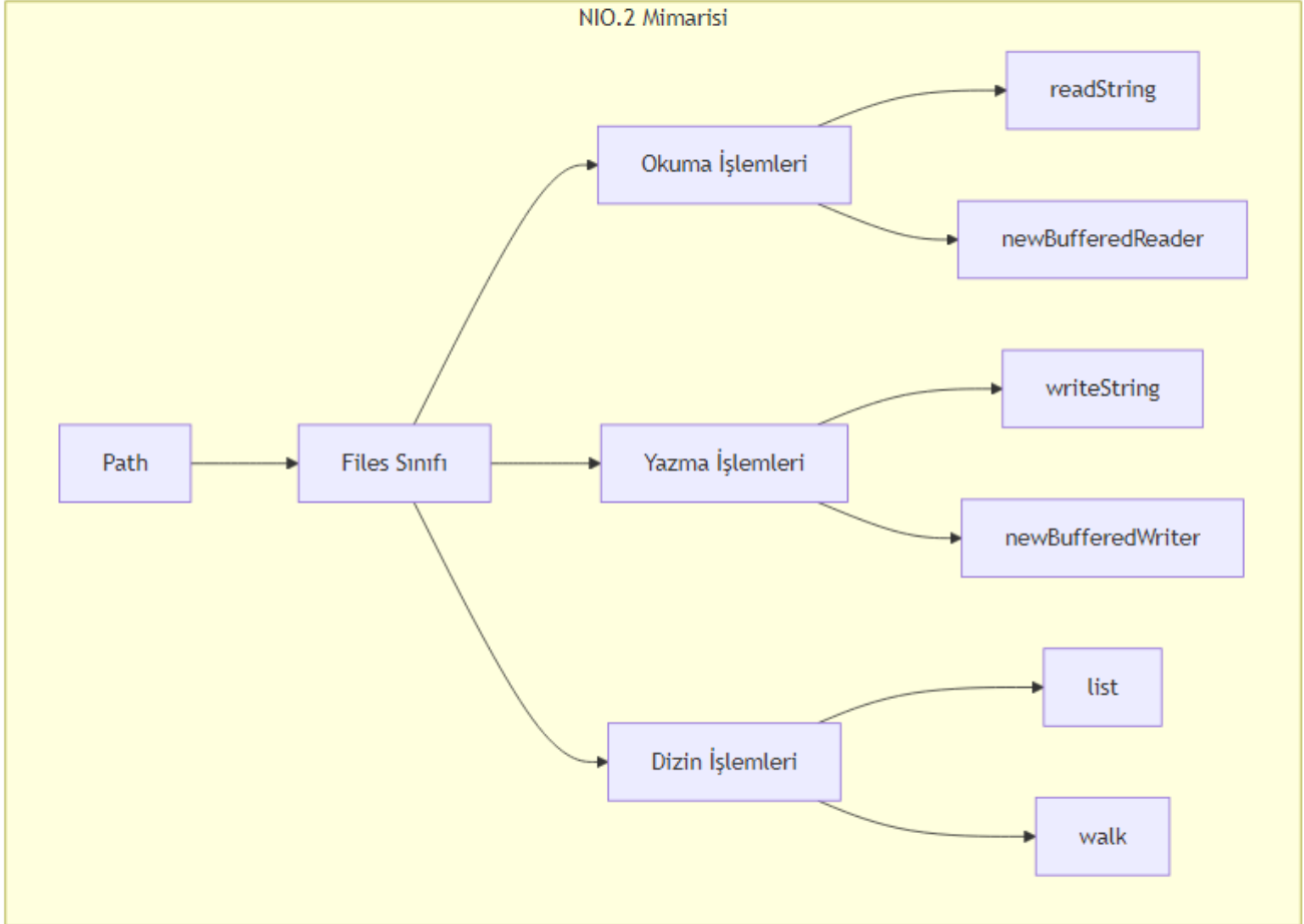
Şekil 20: Mermaid Diyagramı 24
