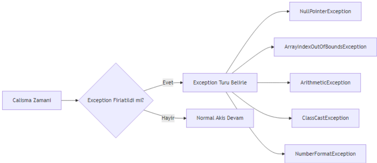
Şekil 44: Mermaid Diyagramı 50
