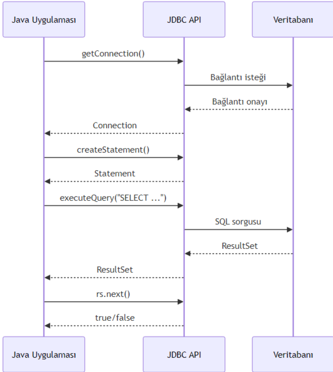
Şekil 39: Mermaid Diyagramı 45
