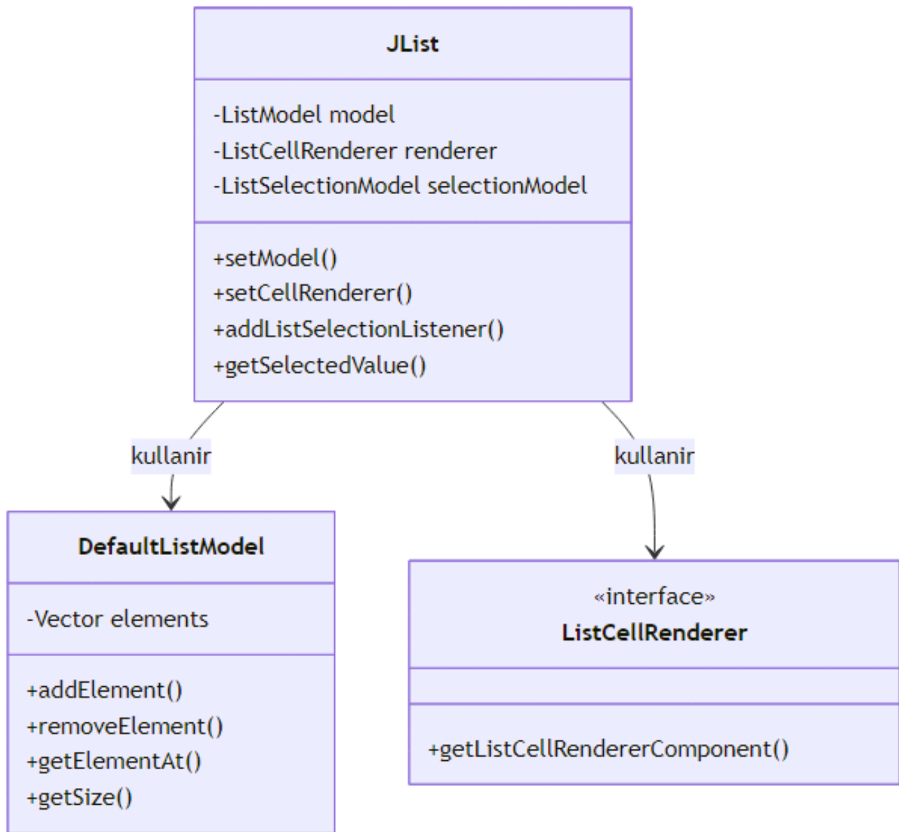
Şekil 34: Mermaid Diyagramı 40
