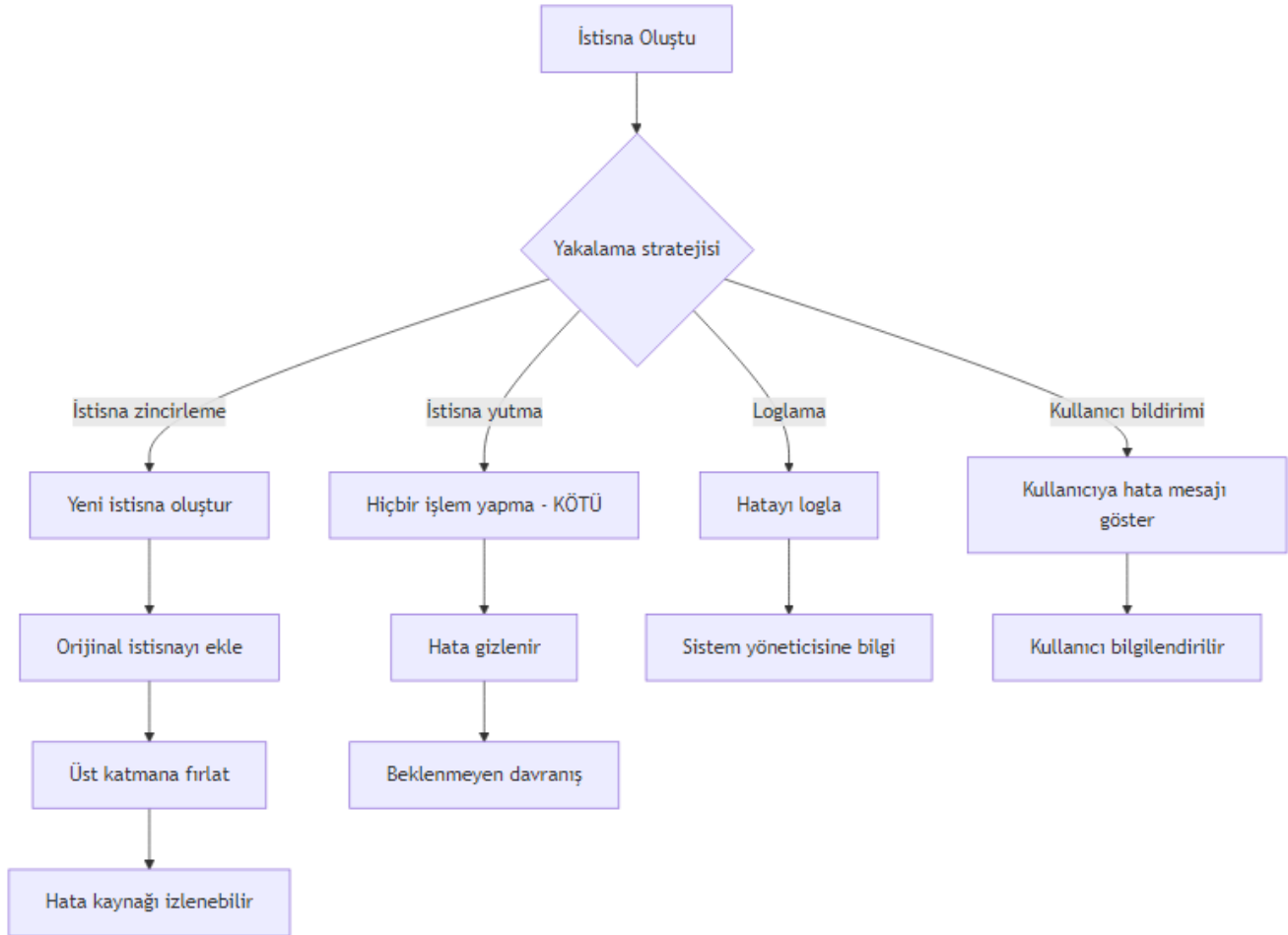
Şekil 17: Mermaid Diyagramı 20
