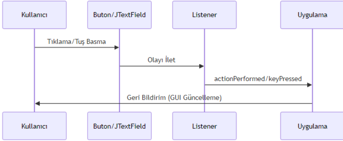
Şekil 32: Mermaid Diyagramı 38
