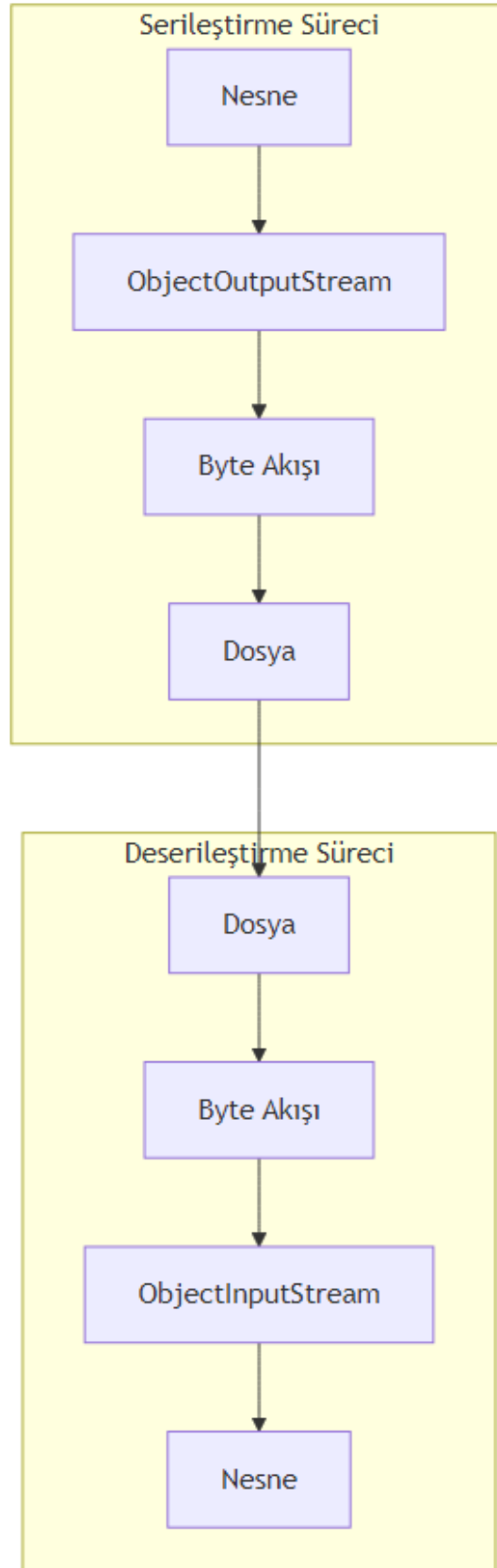
Şekil 21: Mermaid Diyagramı 25
