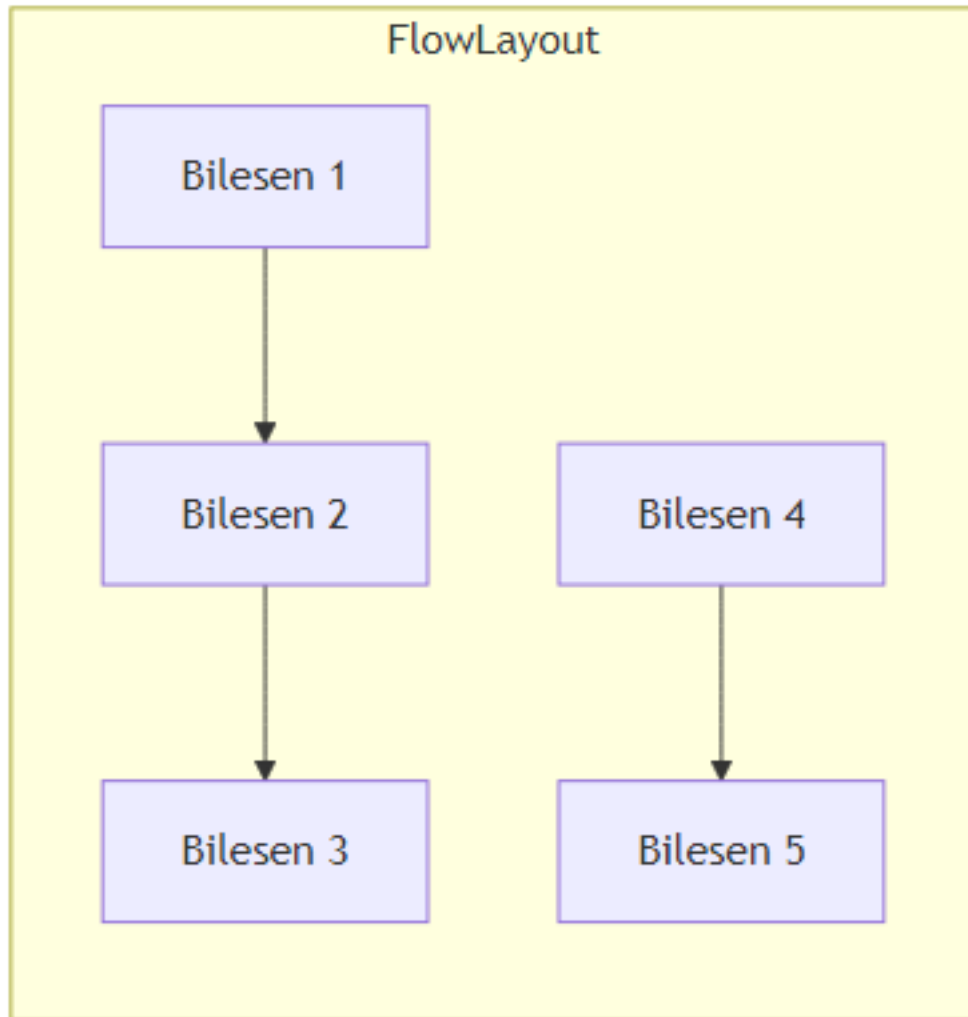
Şekil 28: Mermaid Diyagramı 34
