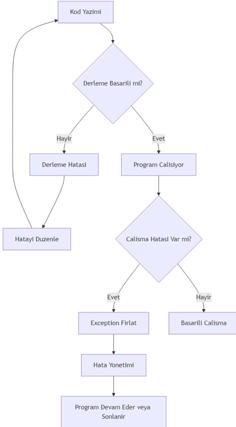
Şekil 43: Mermaid Diyagramı 49
