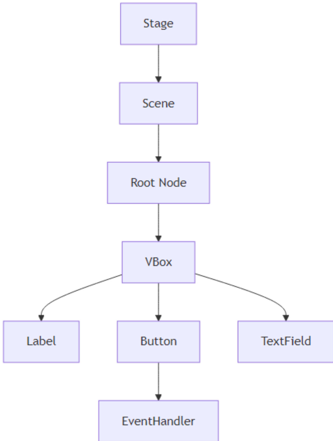
Şekil 46: Mermaid Diyagramı 52
