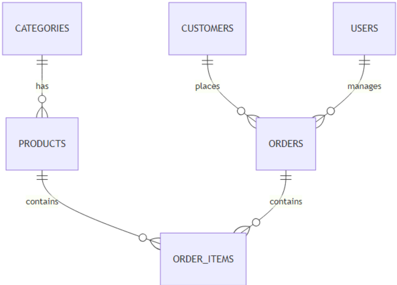
Şekil 42: Mermaid Diyagramı 48
