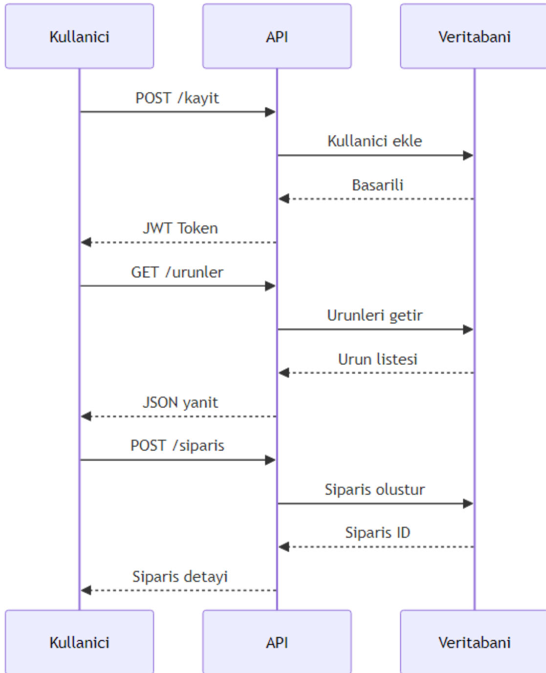
Şekil 50: Mermaid Diyagramı 56
