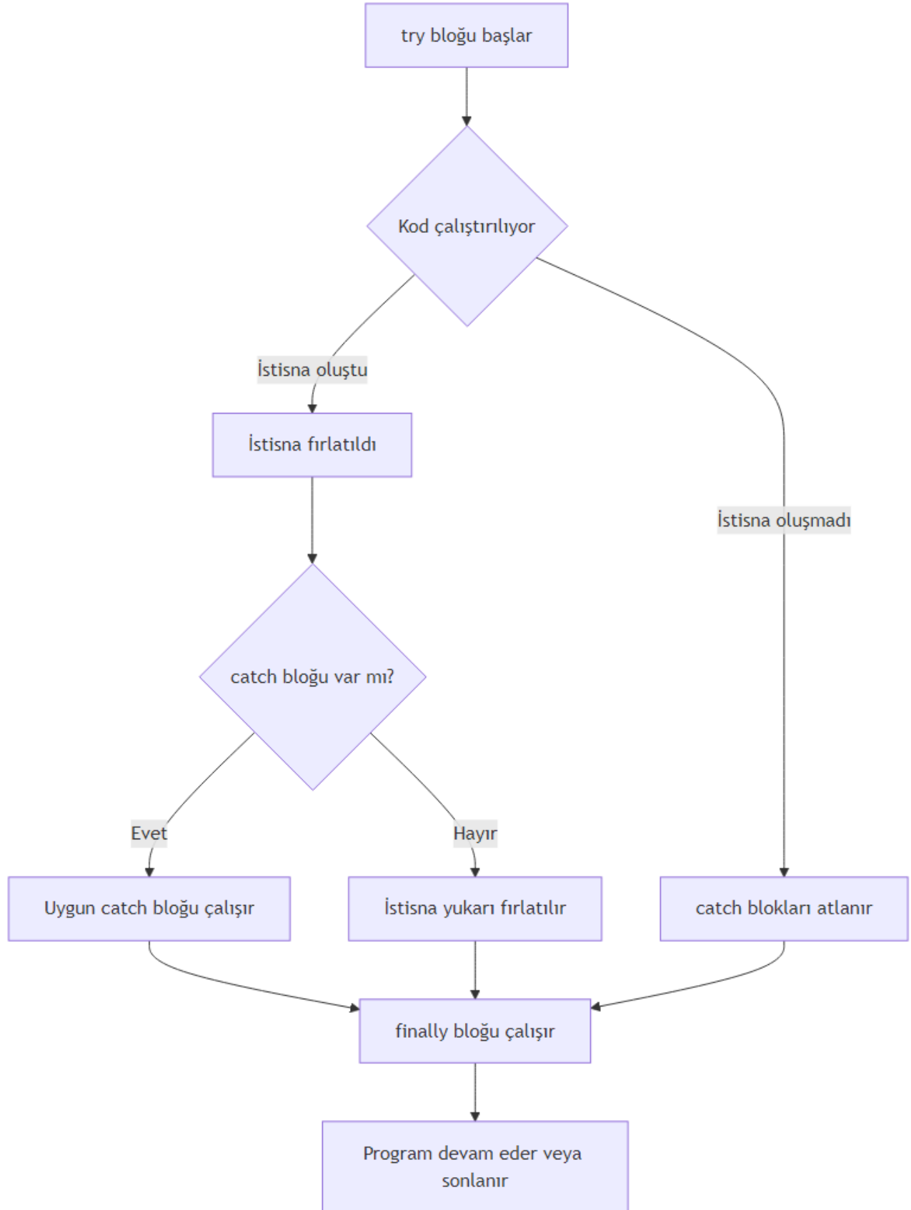
Şekil 14: Mermaid Diyagramı 17
