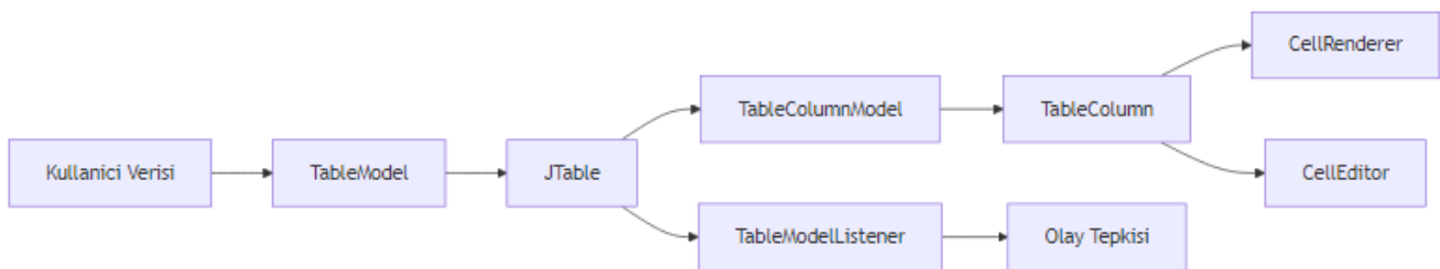
Şekil 35: Mermaid Diyagramı 41
