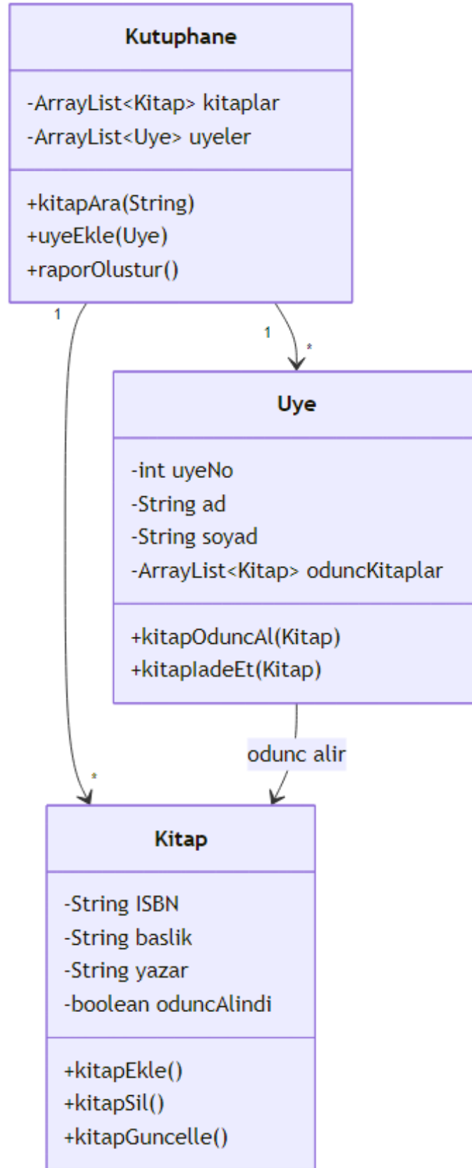
Şekil 49: Mermaid Diyagramı 55
