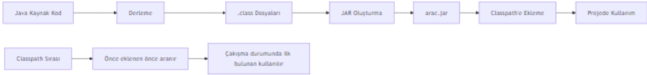
Şekil 8: Mermaid Diyagramı 11
