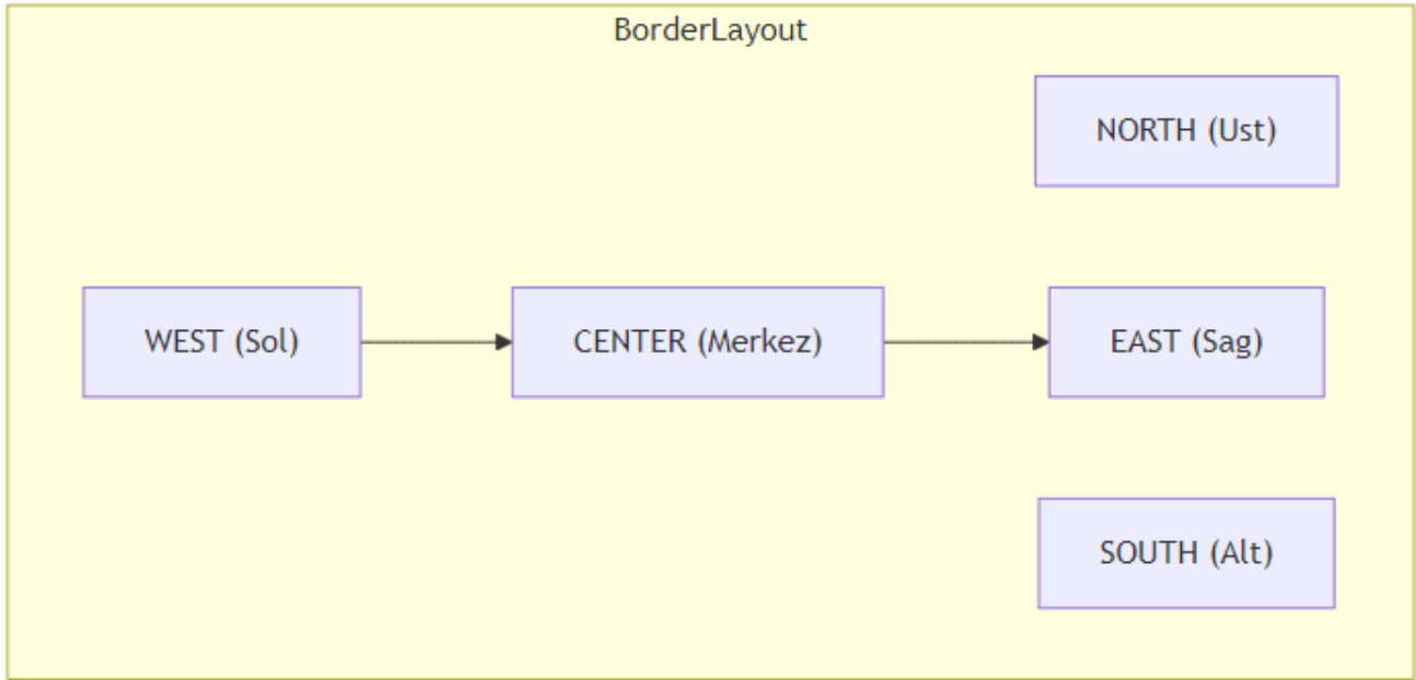
Şekil 29: Mermaid Diyagramı 35
