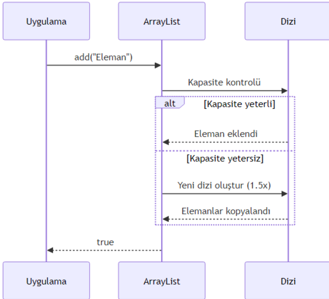
Şekil 10: Mermaid Diyagramı 13
