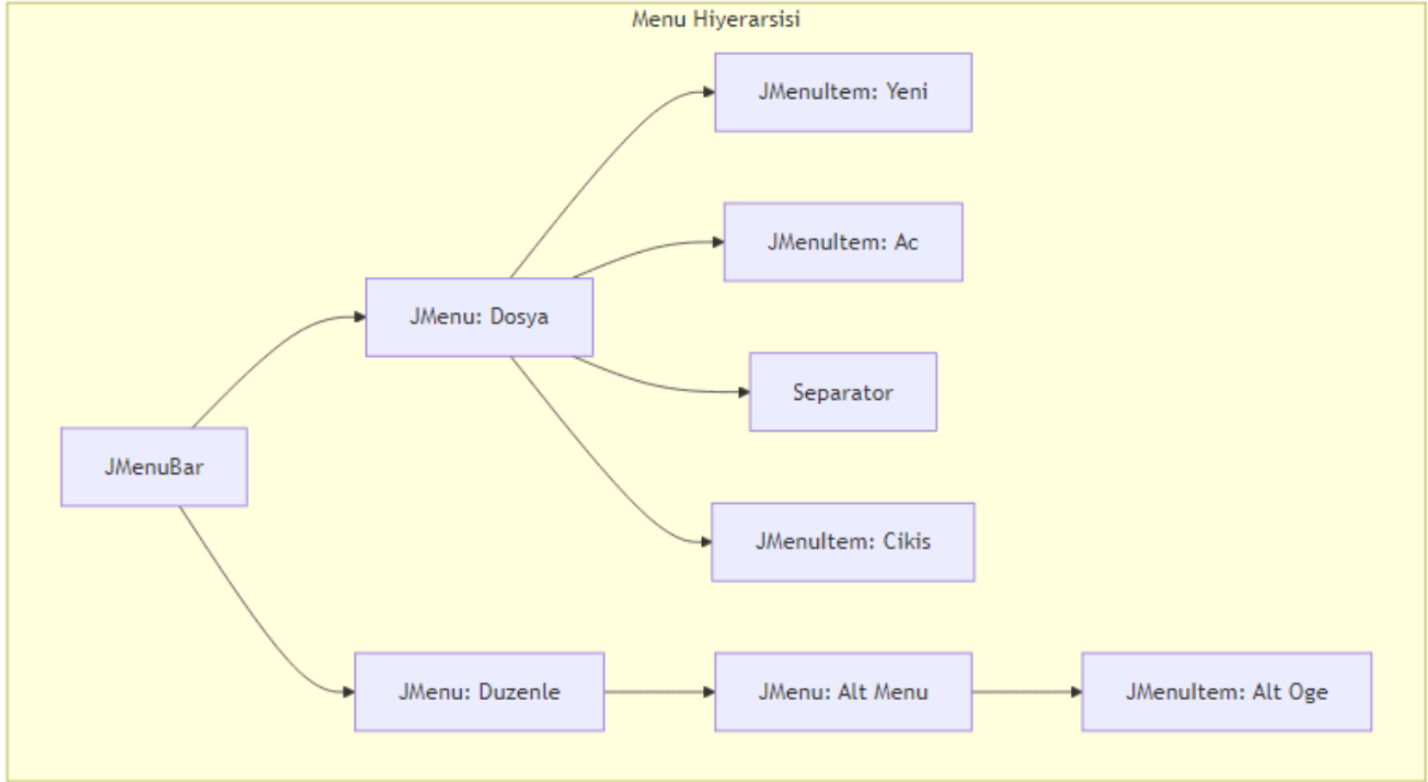
Şekil 36: Mermaid Diyagramı 42
