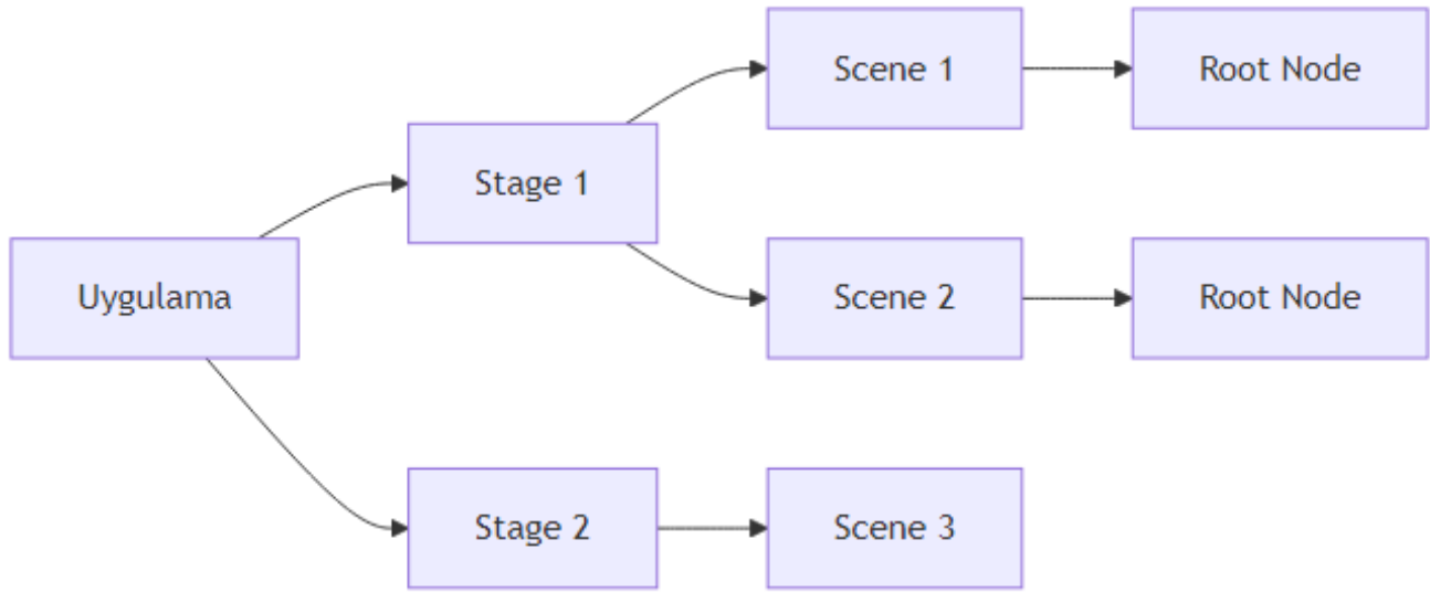
Şekil 47: Mermaid Diyagrami 53
