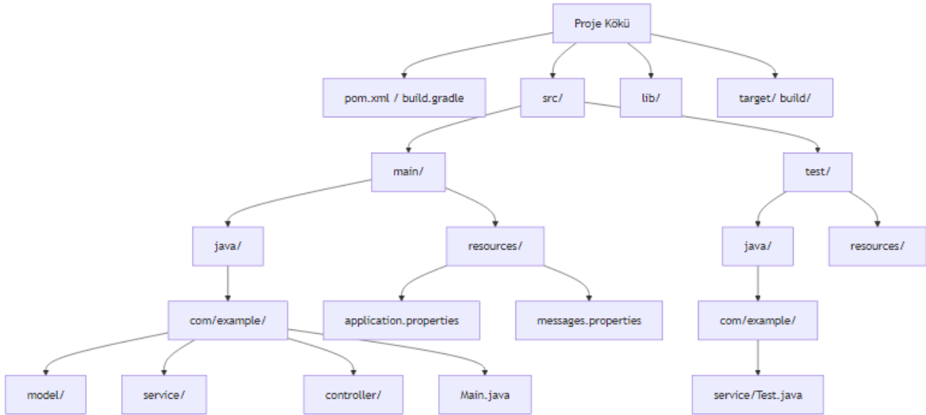
Şekil 7: Mermaid Diyagramı 10
