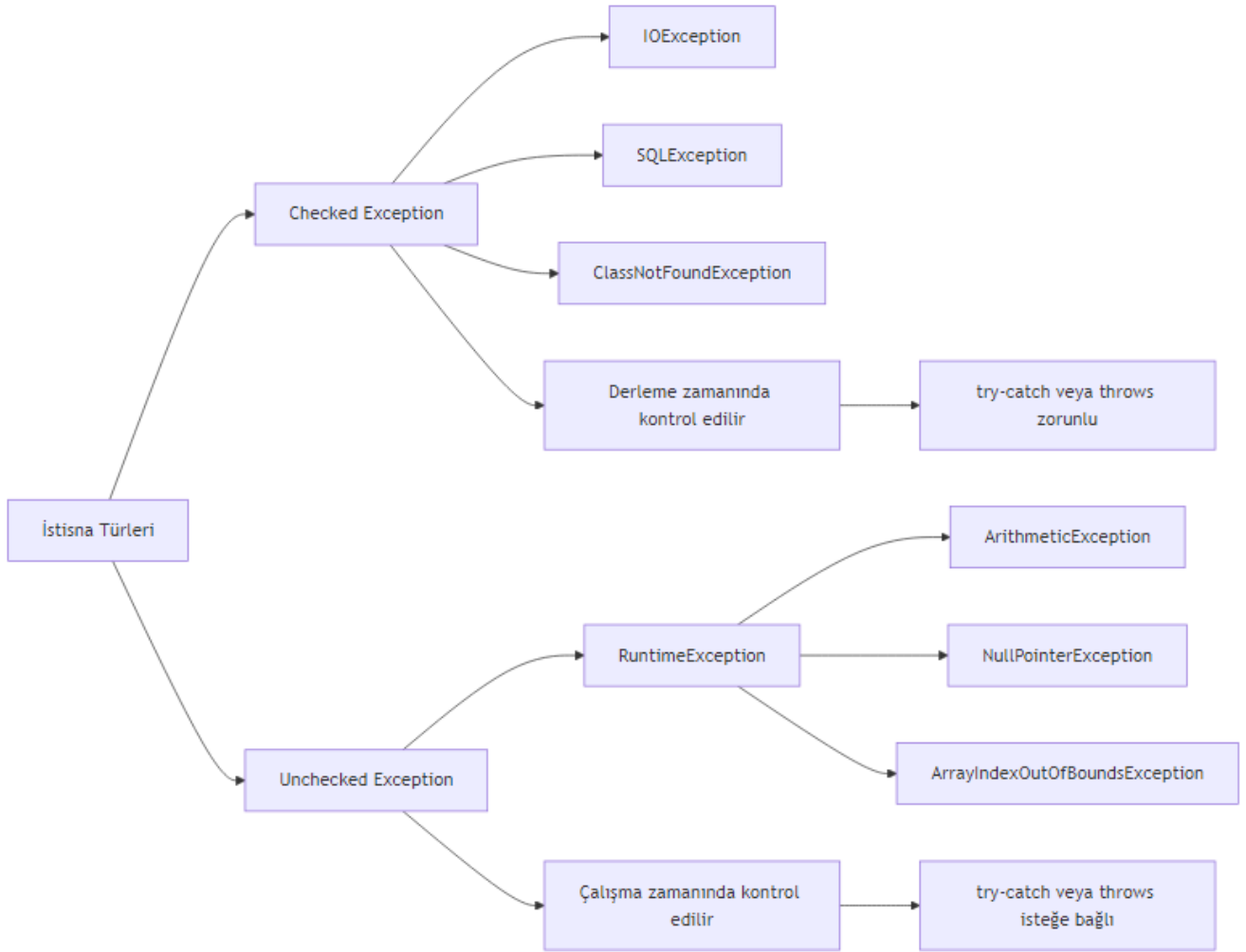
Şekil 15: Mermaid Diyagramı 18
