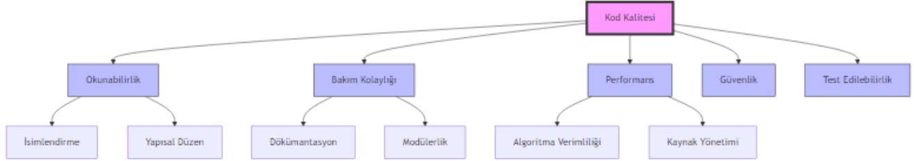
Şekil 51: Mermaid Diyagramı 57
