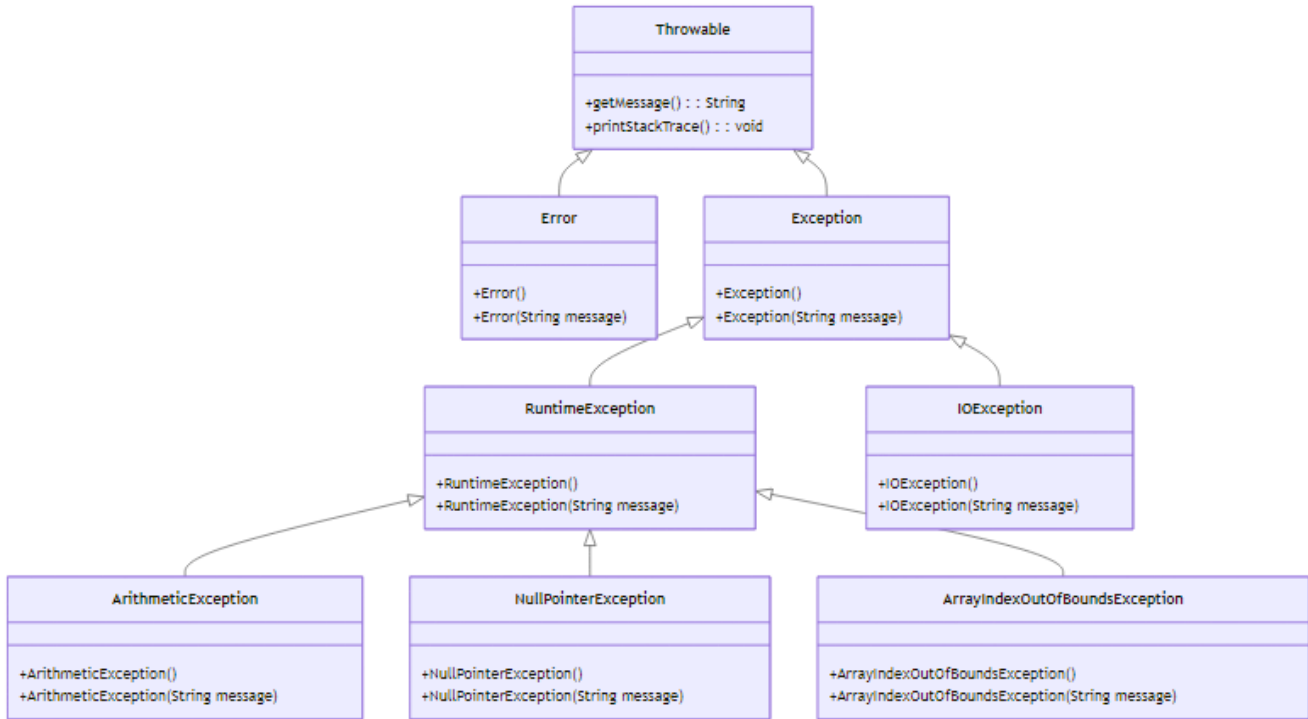
Şekil 13: Mermaid Diyagramı 16
