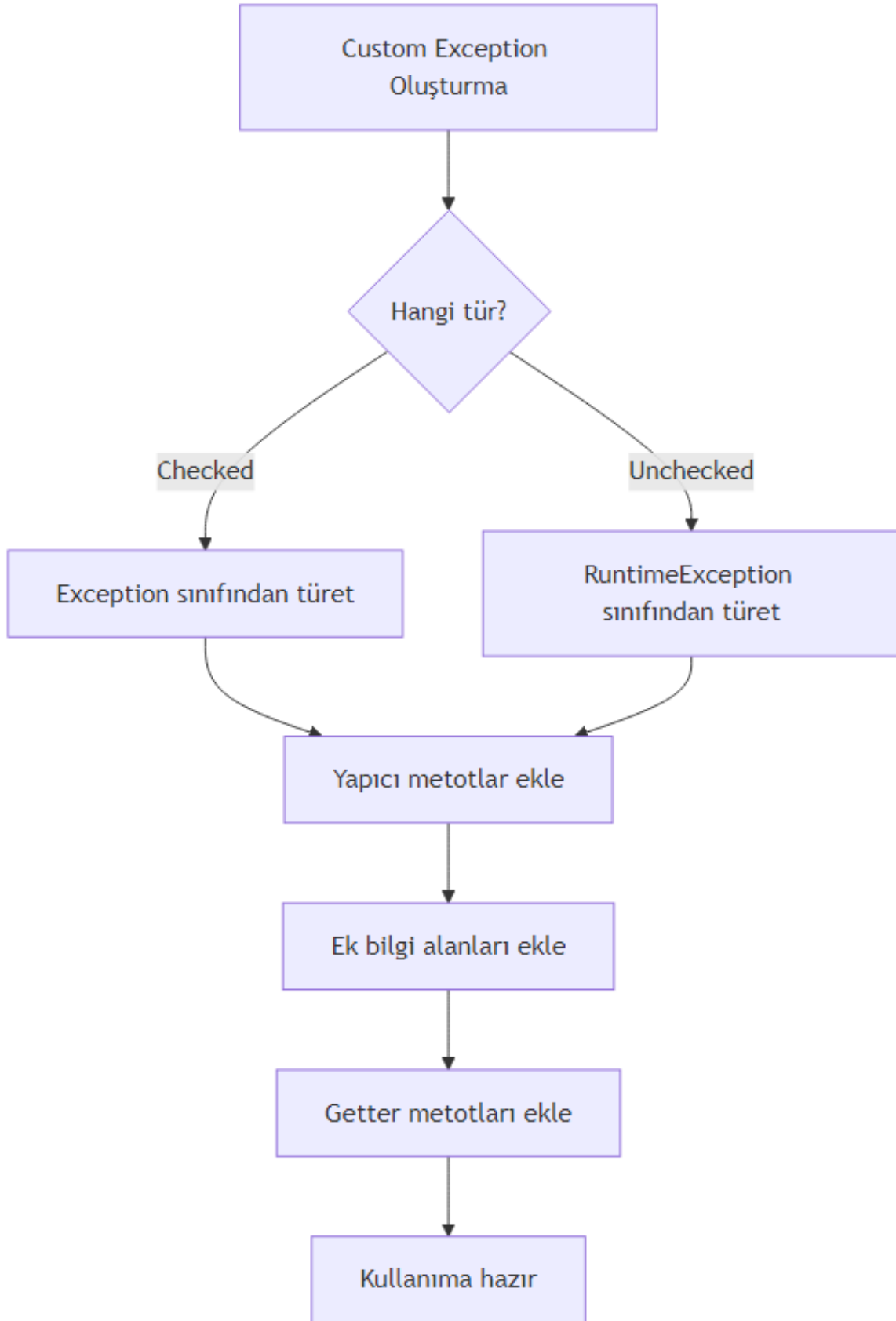
Şekil 16: Mermaid Diyagramı 19
