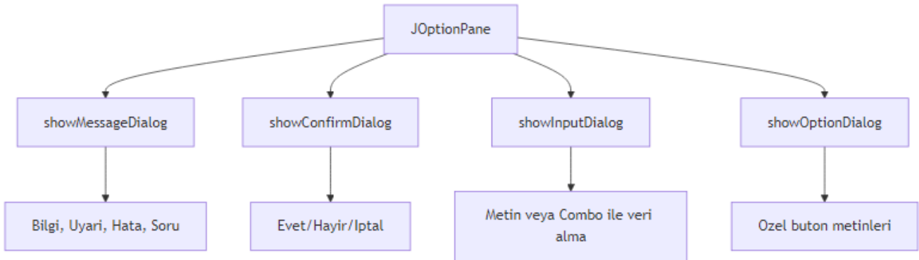
Şekil 37: Mermaid Diyagramı 43
