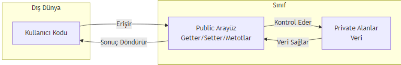
Şekil 22: Mermaid Diyagramı 27
