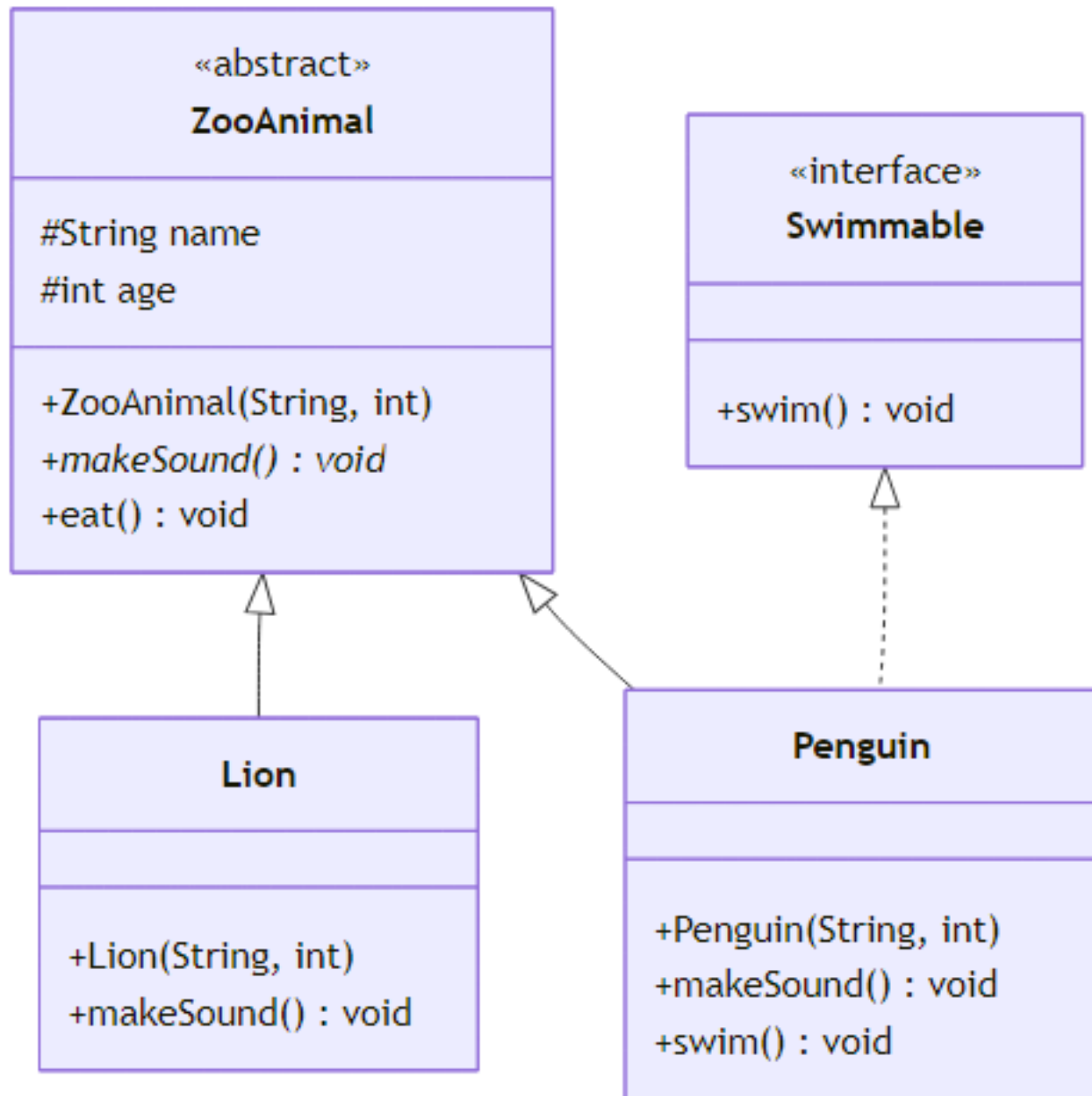
Şekil 26: Mermaid Diyagramı 32
