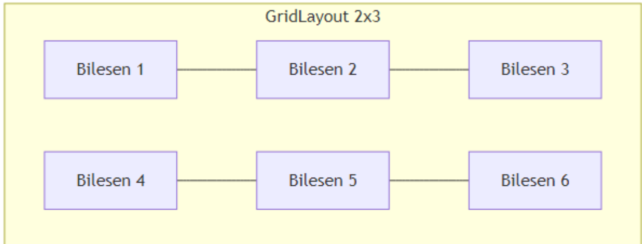
Şekil 30: Mermaid Diyagramı 36
