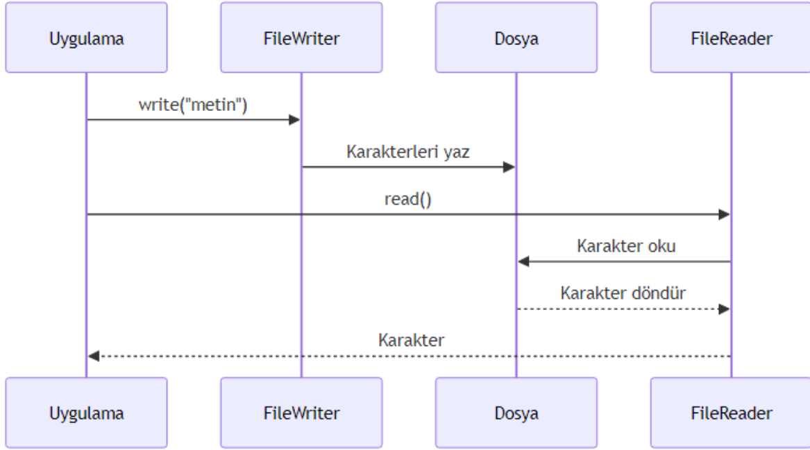
Şekil 18: Mermaid Diyagramı 22
