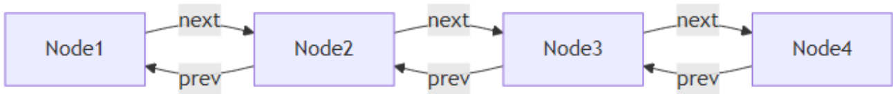
Şekil 11: Mermaid Diyagramı 14
