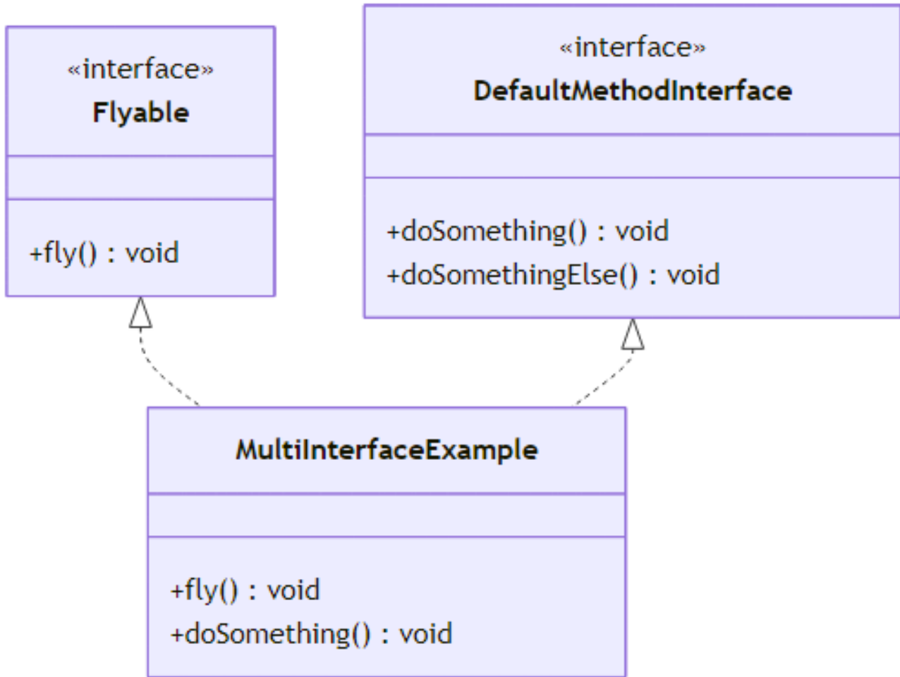
Şekil 25: Mermaid Diyagramı 30
