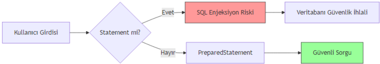
Şekil 40: Mermaid Diyagramı 46
