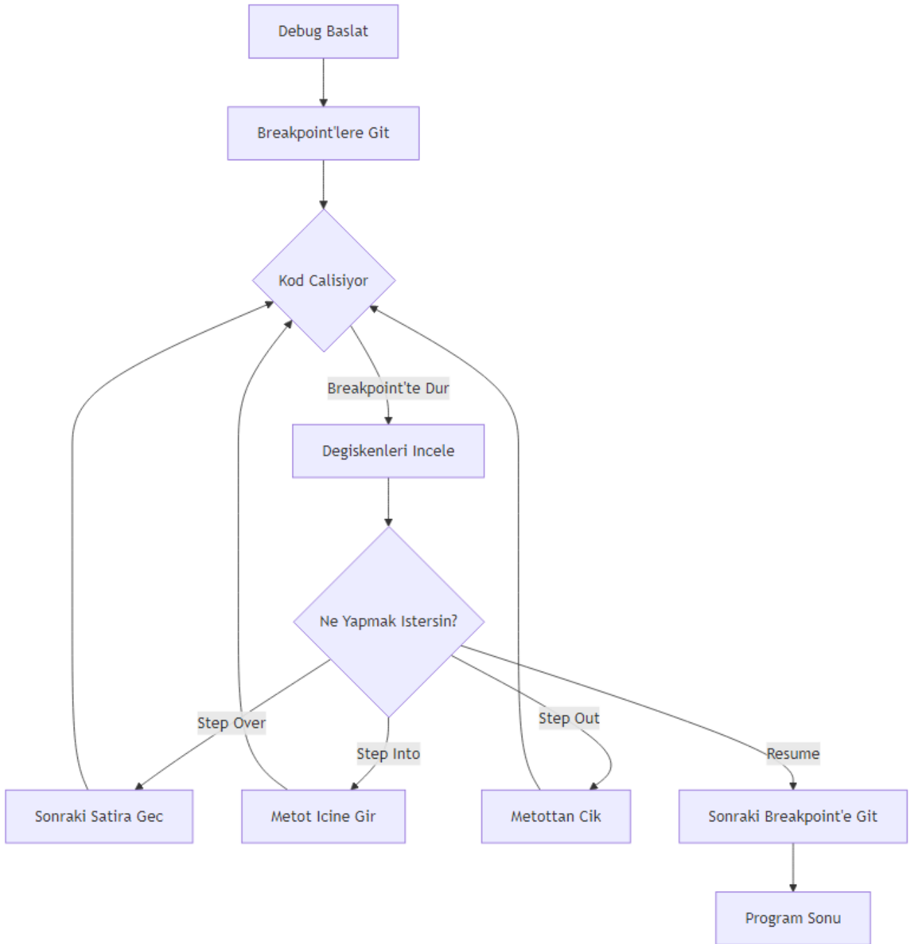
Şekil 45: Mermaid Diyagramı 51
