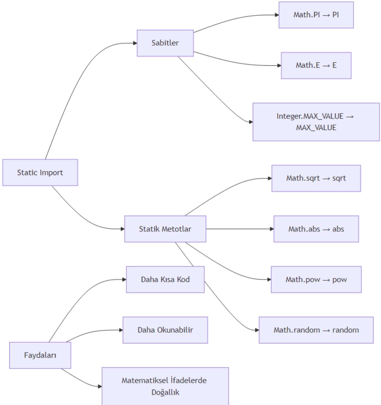
Şekil 6: Mermaid Diyagramı 9
