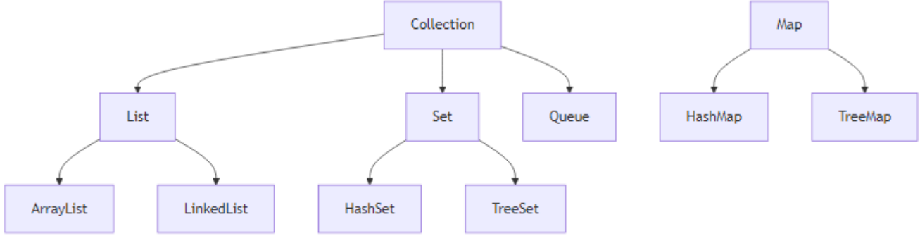
Şekil 9: Mermaid Diyagramı 12
