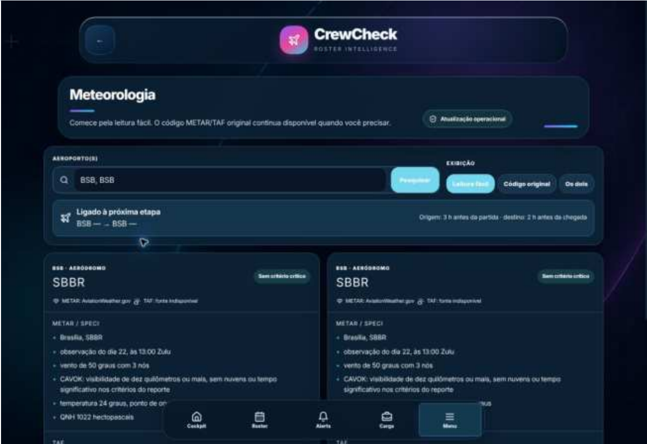
Figura. Meteorologia em cards legíveis, com consulta, formato de exibição e vínculo à próxima etapa.
