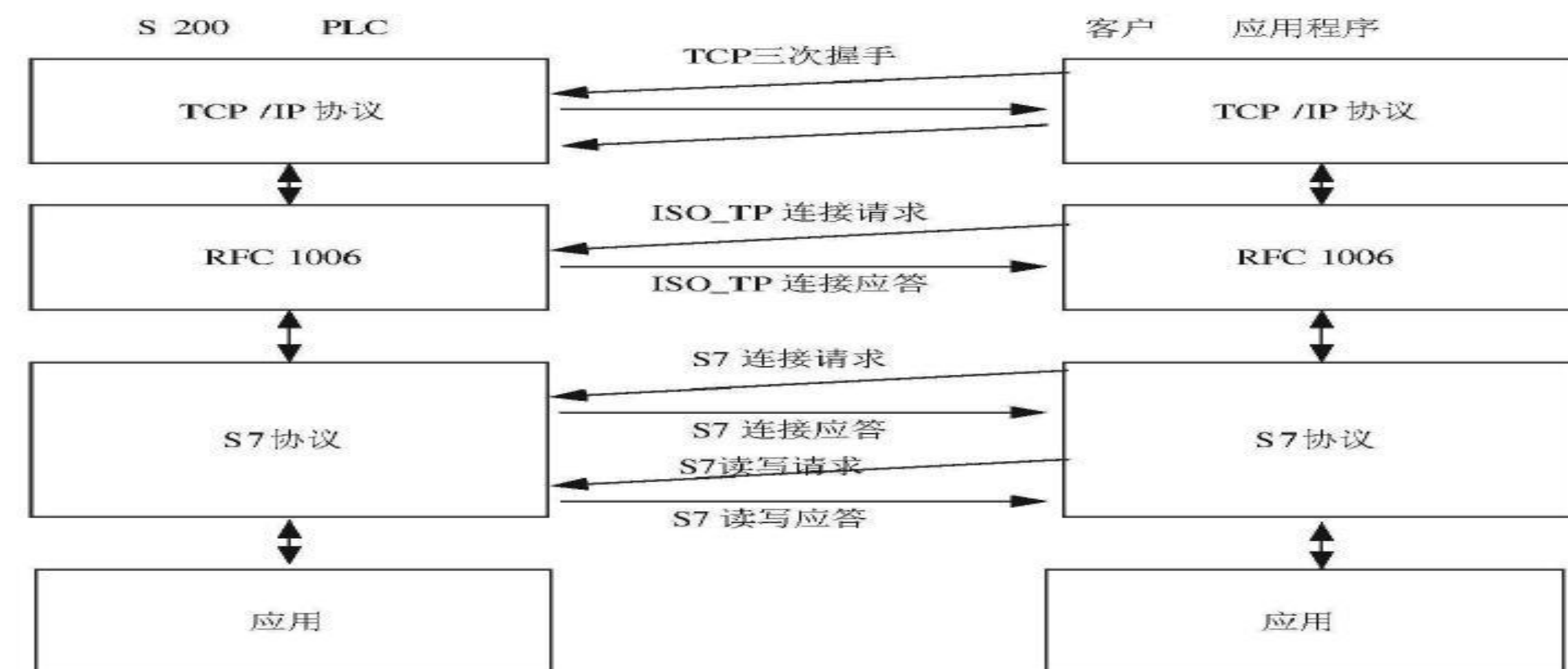
图 2: S7-200 网络通讯过程
