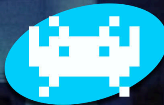
Account-Bot
