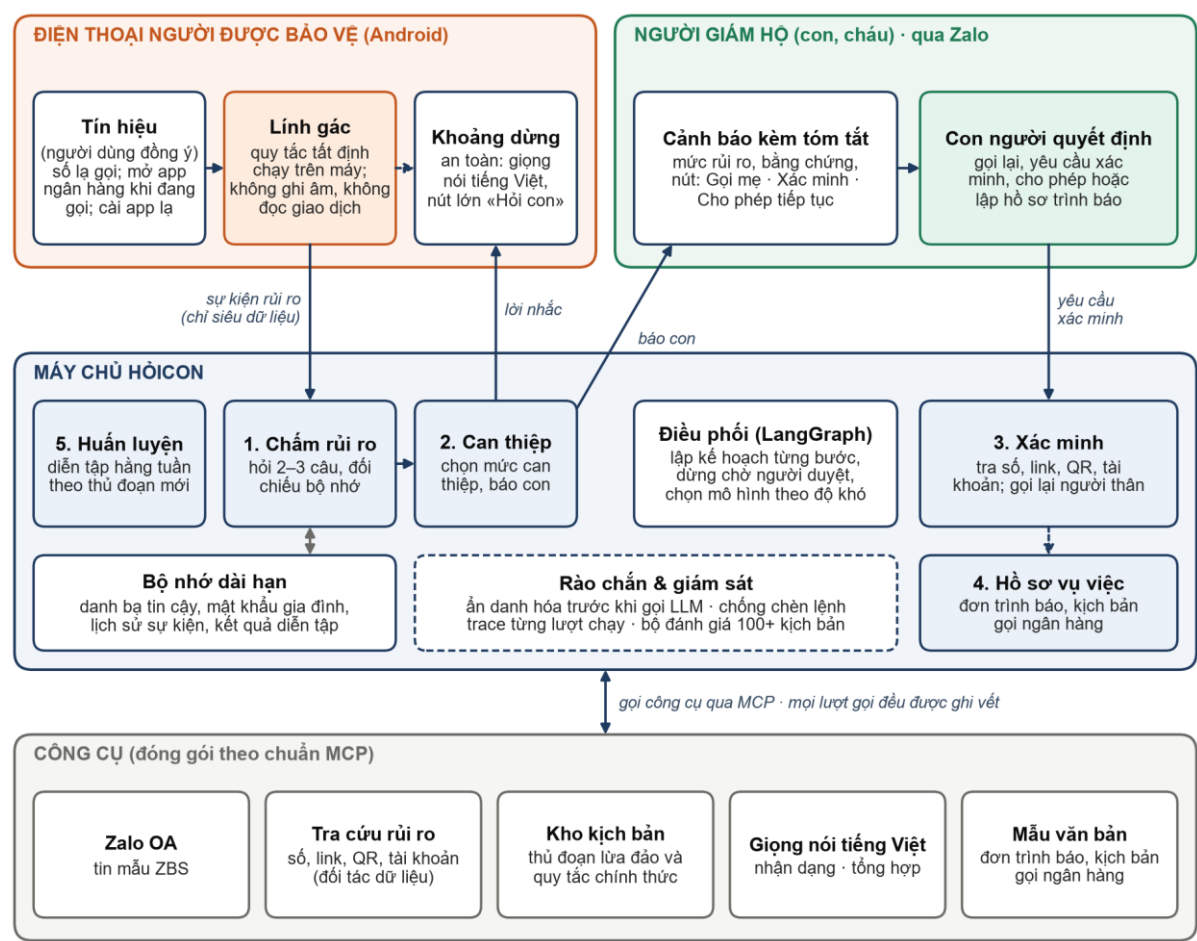
Hình 2. Kiến trúc hệ đa tác tử của HỏiCon
