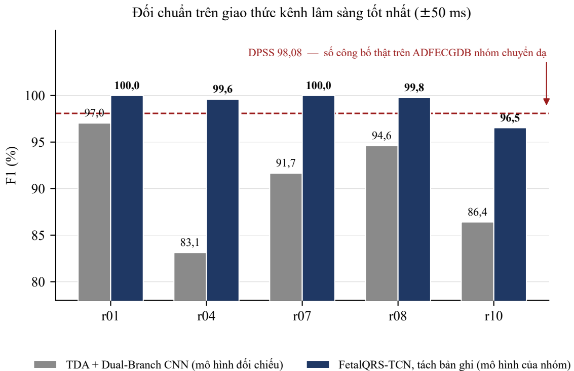
Hình 9: Đối chuẩn trên giao thức kênh lâm sàng tốt nhất, dung sai \pm 50 ms. Đường đứt đỏ là con số thật mà bài DPSS công bố cho nhóm chuyển dạ.
