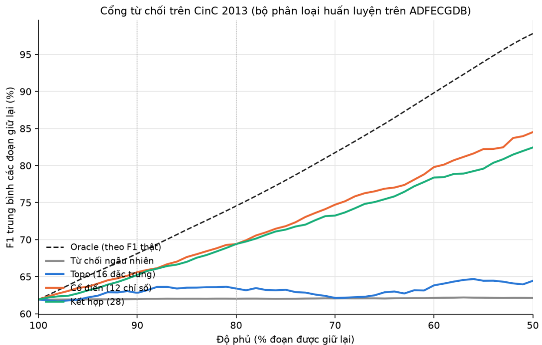
Hình 10: Đường cong rủi ro–độ phủ trên CinC 2013. Đường topo (xanh dương) gần như nằm sát đường từ chối ngẫu nhiên (xám) trên toàn bộ dải độ phủ. Đường cổ điển (cam) tách rõ và tiến về oracle (đứt).
