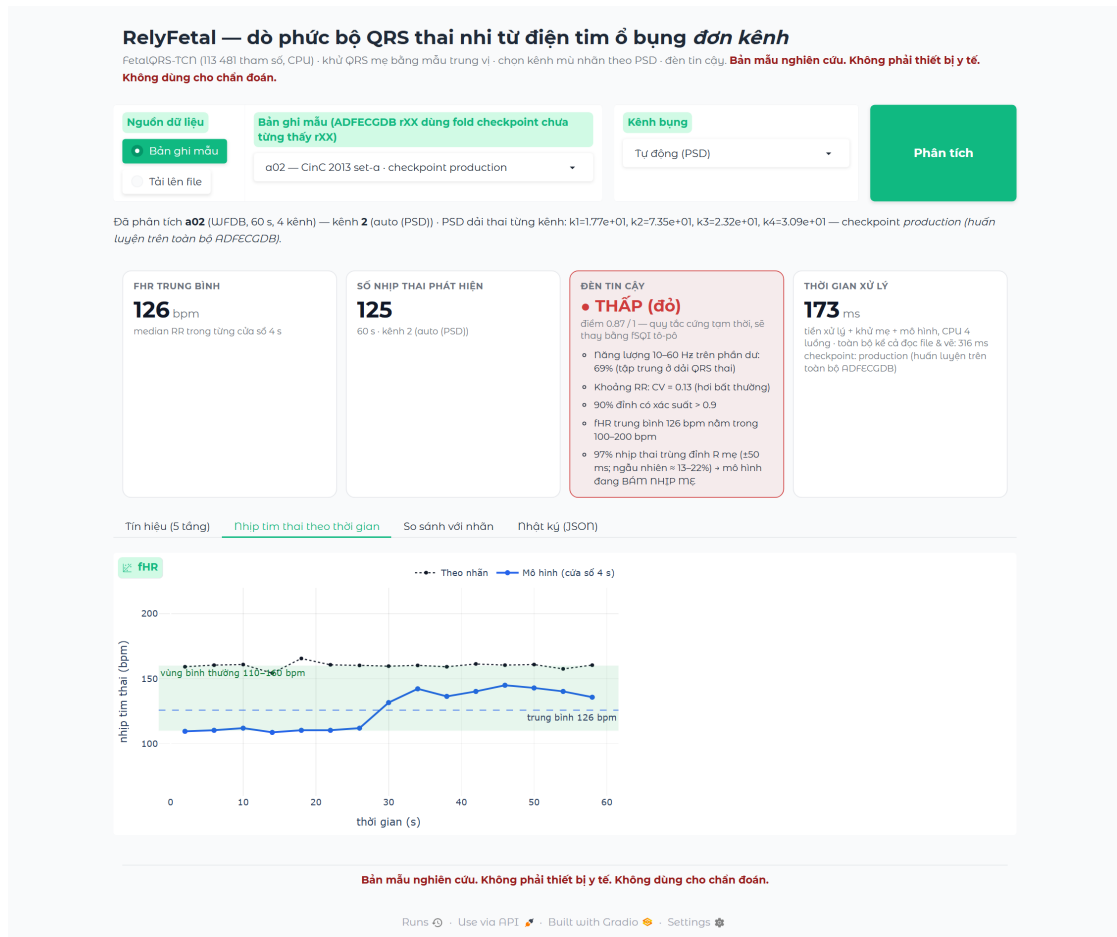
Hình 13: Ảnh chụp trên a02, bản ghi tệ nhất của CinC 2013, zero-shot. Đèn đỏ vì 97% nhịp “thai” trùng đỉnh R mẹ. Đồ thị nhịp tim cho thấy đúng cơ chế thất bại: đường mô hình bám ở nhịp mẹ ( \approx 126 ) trong khi nhãn ở \approx 160 nhịp/phút. Hệ thống tự phát hiện và từ chối, thay vì báo sai.
