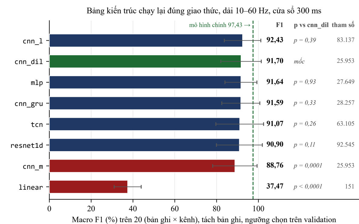
Hình 3: Tám kiến trúc dưới giao thức trung thực. Hiệu số so với cnn_dil nằm trong khoảng -2,95 đến +0,73 điểm; với n = 5 chủ thể nghiên cứu này không đủ lực để kết luận chúng tương đương (§10). Đường đứt xanh là mô hình chính (ngữ cảnh 4 giây, đầu ra từng mẫu) — cách xa cả nhóm.
