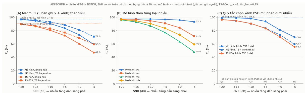
Hình 11: (A) Macro F1 theo SNR, mô hình so với TS-PCA, nhiễu hỗn hợp và trung bình ba loại. (B) Mô hình theo từng loại nhiễu: trôi nền gần như vô hại, nhiễu cơ hại nhất. (C) Quy tắc chọn kênh PSD mũ nhân dưới nhiễu, kèm số bản ghi giữ nguyên kênh đã chọn so với khi không nhiễu.
