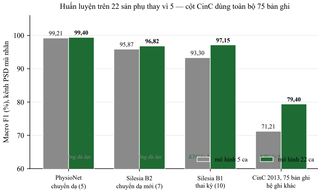
Hình 12: Cùng chủ thể, cùng giao thức, chỉ đổi mô hình. Cột CinC 2013 trong hình vẽ trên 75 bản ghi (đã rút ở bản 3.5; số đúng trên 60 bản sạch là 64,04 → 74,28, §5.10.3); bản 3.2 dùng 90,34 — kênh 0 hậu kiểm trên 10 bản ghi, cũng đã rút. Lợi ích tập trung đúng ở hai chỗ yếu: thai kỳ và hệ ghi khác; hai nhóm bên trái có n quá nhỏ để kết luận.
