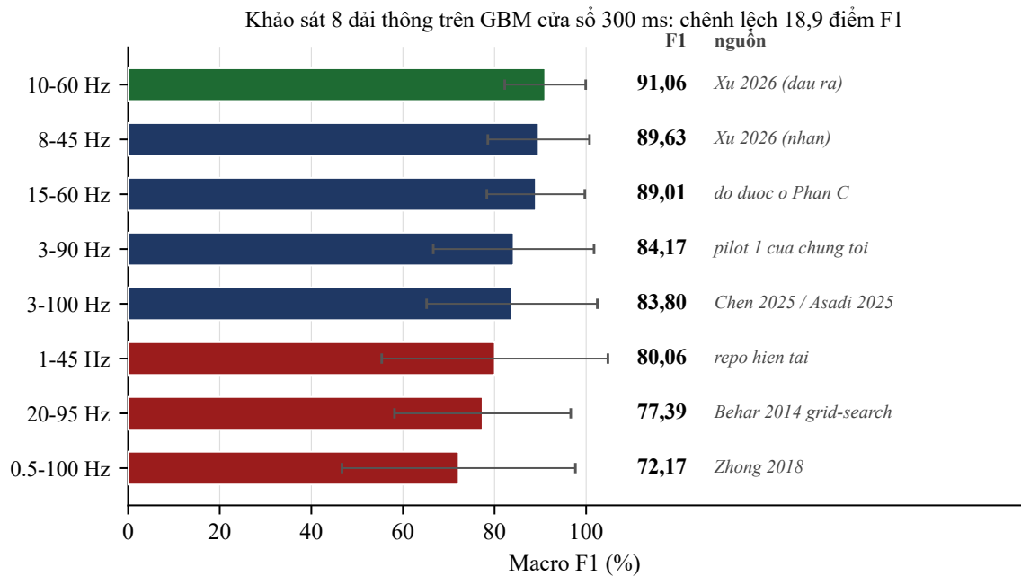
Hình 7: Khảo sát tám dải thông trên gradient boosting , cửa sổ 300 ms , mỗi dải là một lần chạy tách theo bản ghi đầy đủ. Chênh lệch giữa dải tốt nhất và kém nhất là 18,89 điểm F1 — lớn hơn toàn bộ khác biệt giữa 16 kiến trúc học sâu. Cảnh báo phạm vi: độ lớn này không chuyển sang TCN — xem §5.2.1.
