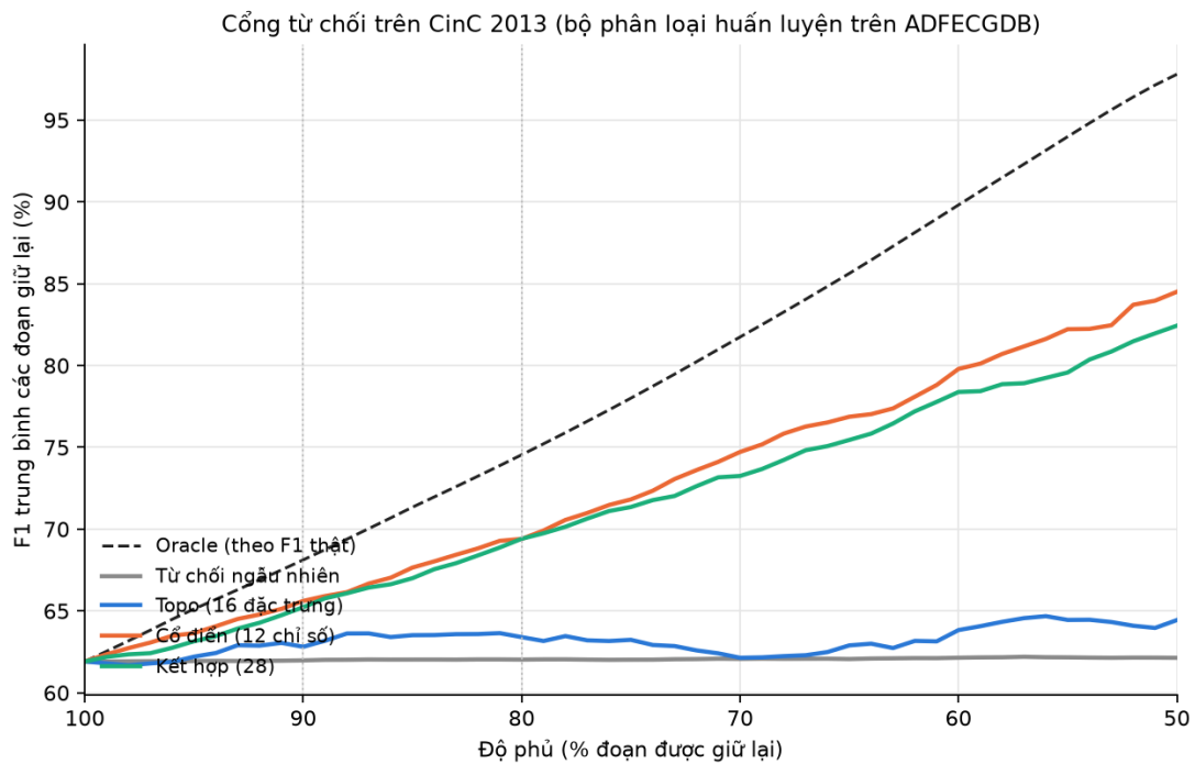
Hình 16: Đường cong rủi ro–độ phủ trên CinC 2013. Đường topo (xanh dương) gần như nằm sát đường từ chối ngẫu nhiên (xám) trên toàn bộ dải độ phủ. Đường cổ điển (cam) tách rõ và tiến về oracle (đứt).
