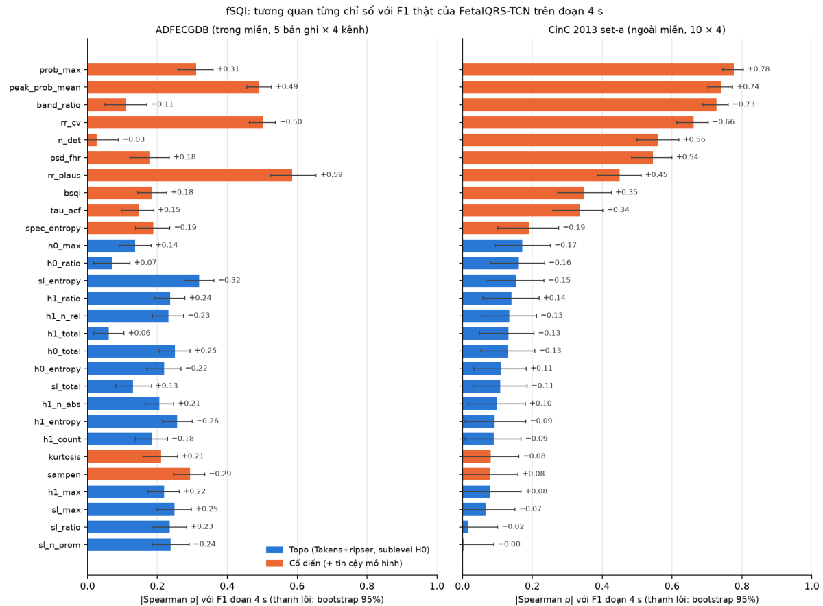
Hình 17: Tương quan Spearman của từng chỉ số với F1 đoạn, kèm khoảng tin cậy bootstrap 95%. Trái: trong miền. Phải: ngoài miền. Các chỉ số cổ điển (cam) mạnh lên khi ra ngoài miền; các chỉ số topo (xanh) yếu đi và nhiều chỉ số đổi dấu.
