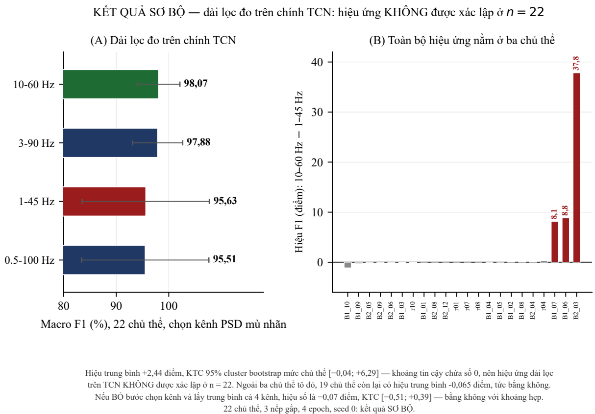
Hình 8: Dải lọc đo trên chính TCN, cả bốn dải. (A) macro F1 theo quy tắc chọn kênh PSD mù nhãn. (B) hiệu số từng chủ thể giữa 10–60 Hz và 1–45 Hz: 19 trong 22 chủ thể nằm sát số không, toàn bộ hiệu ứng do ba chủ thể tô đỏ tạo ra. Dòng chú dưới hình ghi thêm kết quả trên thang đo trung bình 4 kênh , nơi hiệu số bằng không với khoảng hẹp.
