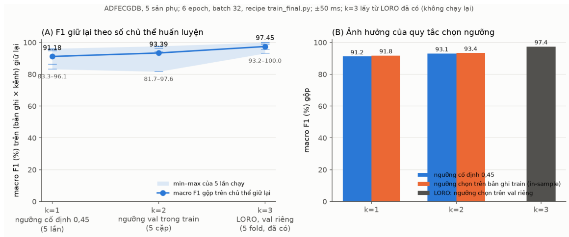
Hình 14: (A) Macro F1 trên chủ thể giữ lại theo số chủ thể huấn luyện; dải mờ là min-max của 5 lần chạy. (B) Ảnh hưởng của quy tắc chọn ngưỡng. Với k = 1 không có chủ thể validation nên dùng ngưỡng cố định 0,45; với k = 2 ngưỡng chọn trên một chủ thể trong tập huấn luyện — cả hai đều được ghi rõ.
