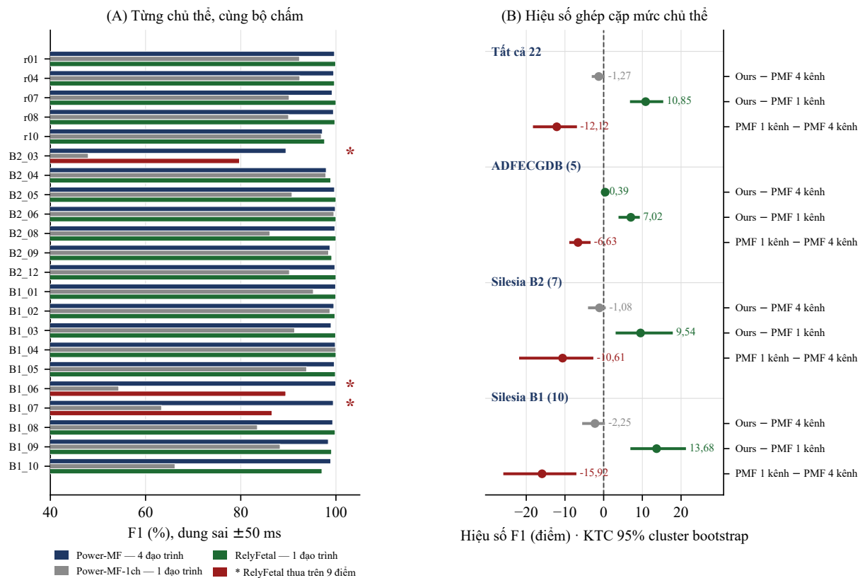
Hình 10: (A) F1 từng chủ thể ở ba cấu hình, cùng bộ chấm \pm 50 ms. Ba chủ thể có dấu sao là ba bản ghi RELYFETAL thua nặng — và Power-MF-1ch cũng sụp ở đúng ba chỗ đó. (B) Hiệu số ghép cặp và KTC 95% cluster bootstrap theo tập con, cho cả ba phép so sánh.
