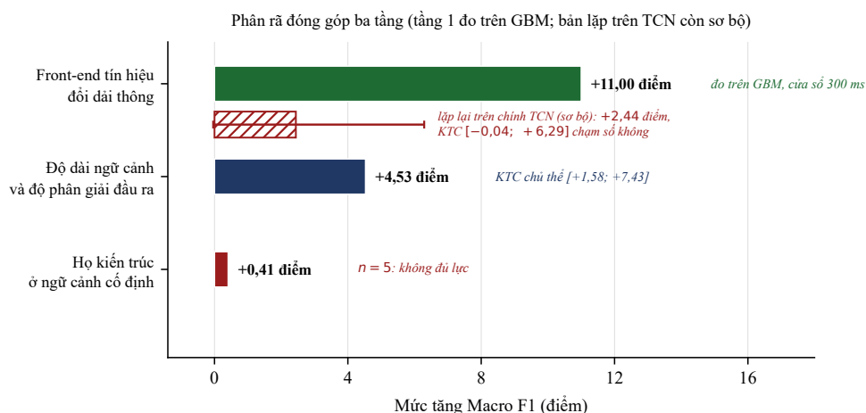
Hình 6: Phân rã đóng góp ba tầng. Trên bộ học cửa sổ 300 ms, front-end tín hiệu vẫn là tầng lớn nhất, và khoảng cách so với tầng ngữ cảnh là 2,4 lần chứ không phải 30 lần như bản đề cương trước phát biểu. Thanh gạch chéo là bản lập lại tầng 1 trên chính TCN : chỉ +2,44 điểm với KTC [-0,04; +6,29] chạm số không — kết quả sơ bộ , xem §5.2.1.
