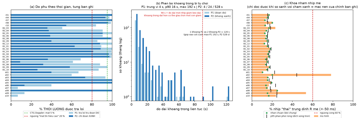
Hình 21: (a) % thời lượng trả lời từng bản ghi so với mốc CTG. (b) Phân bố độ dài khoảng trống, thang log, mốc 90 giây. (c) Khoá nhịp mẹ so với nhãn chuẩn và phân phối rộng.
