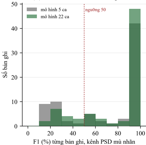
(A) Phân bố trên toàn bộ 75 bản ghi set-a
