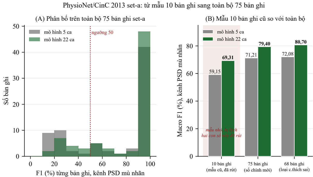
Hình 13: (A) Phân bố F1 từng bản ghi trên toàn bộ 75 bản ghi set-a — vẫn lượng cực : một đỉnh ở 90–100 và một đỉnh dưới 30. Mô hình 22 ca đẩy khối lượng sang phải nhưng không xóa đỉnh thấp. (B) Mẫu 10 bản ghi cũ so với toàn bộ.
