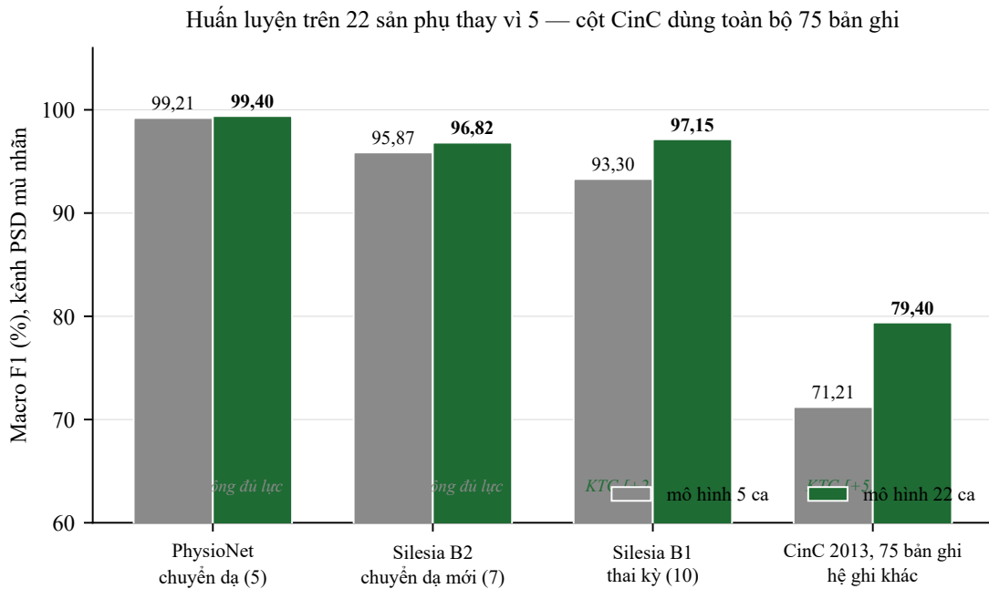
Hình 12: Cùng chủ thể, cùng giao thức, chỉ đổi mô hình. Cột CinC 2013 dùng toàn bộ 75 bản ghi với quy tắc PSD mù nhãn (bản 3.2 dùng 90,34 — kênh 0 hậu kiểm trên 10 bản ghi, đã bị rút). Lợi ích tập trung đúng ở hai chỗ yếu: thai kỳ và hệ ghi khác; hai nhóm bên trái có n quá nhỏ để kết luận.
